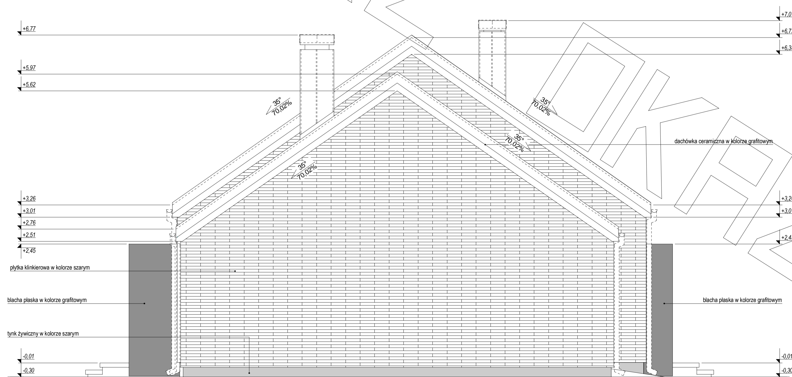
ELEWACJA BOCZNA:
