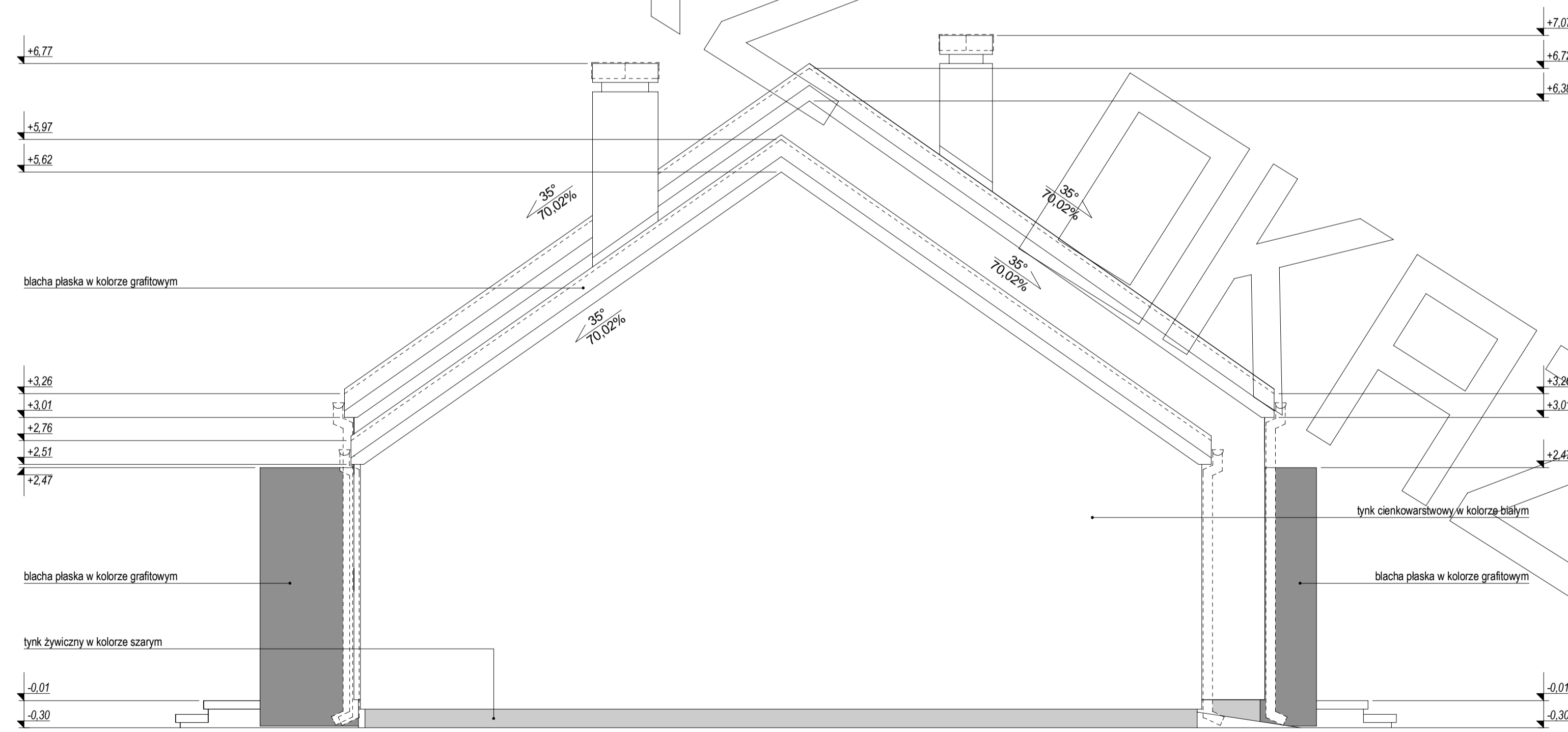
ELEWACJA BOCZNA:
