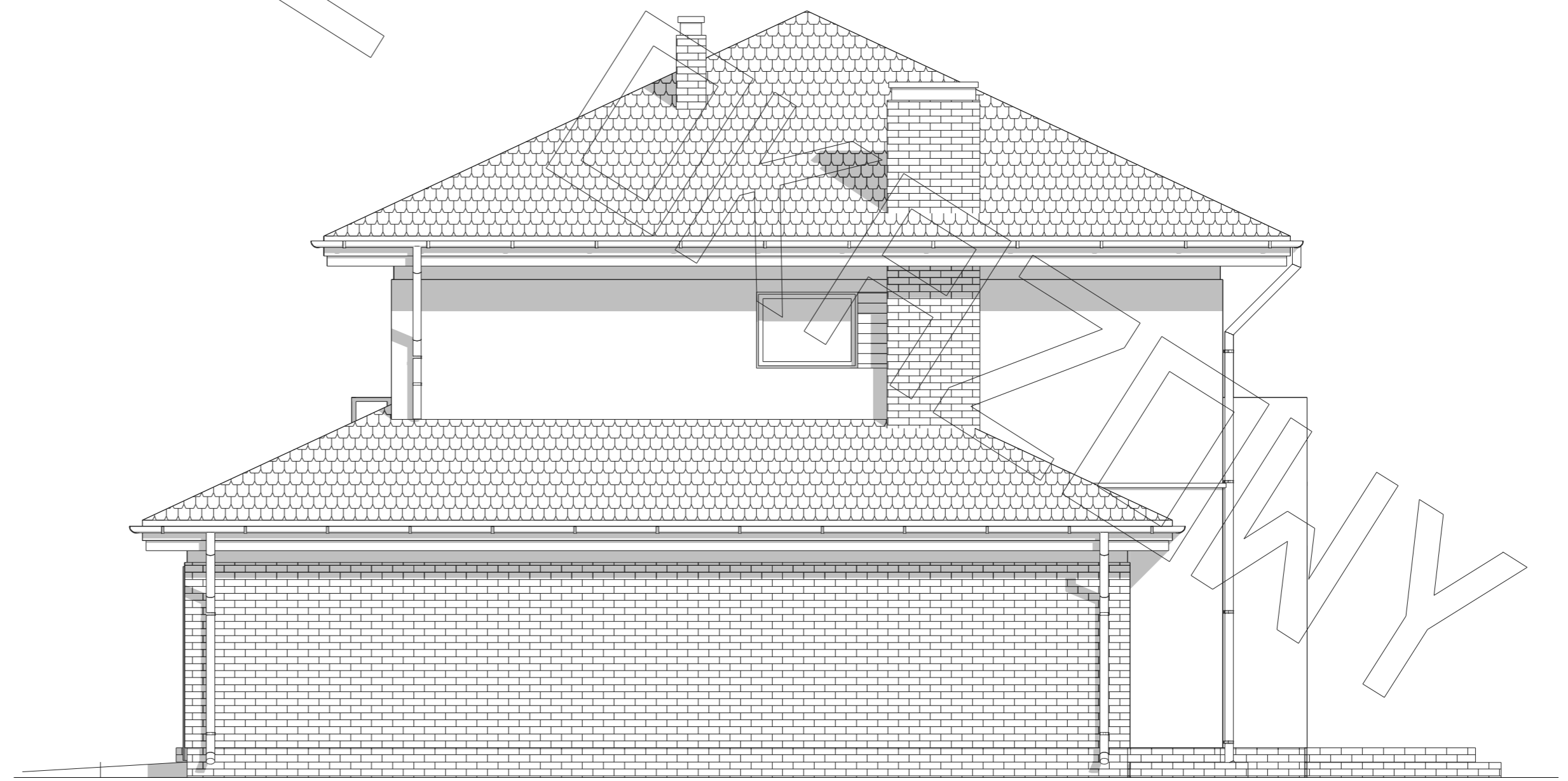
ELEWACJA BOCZNA :
