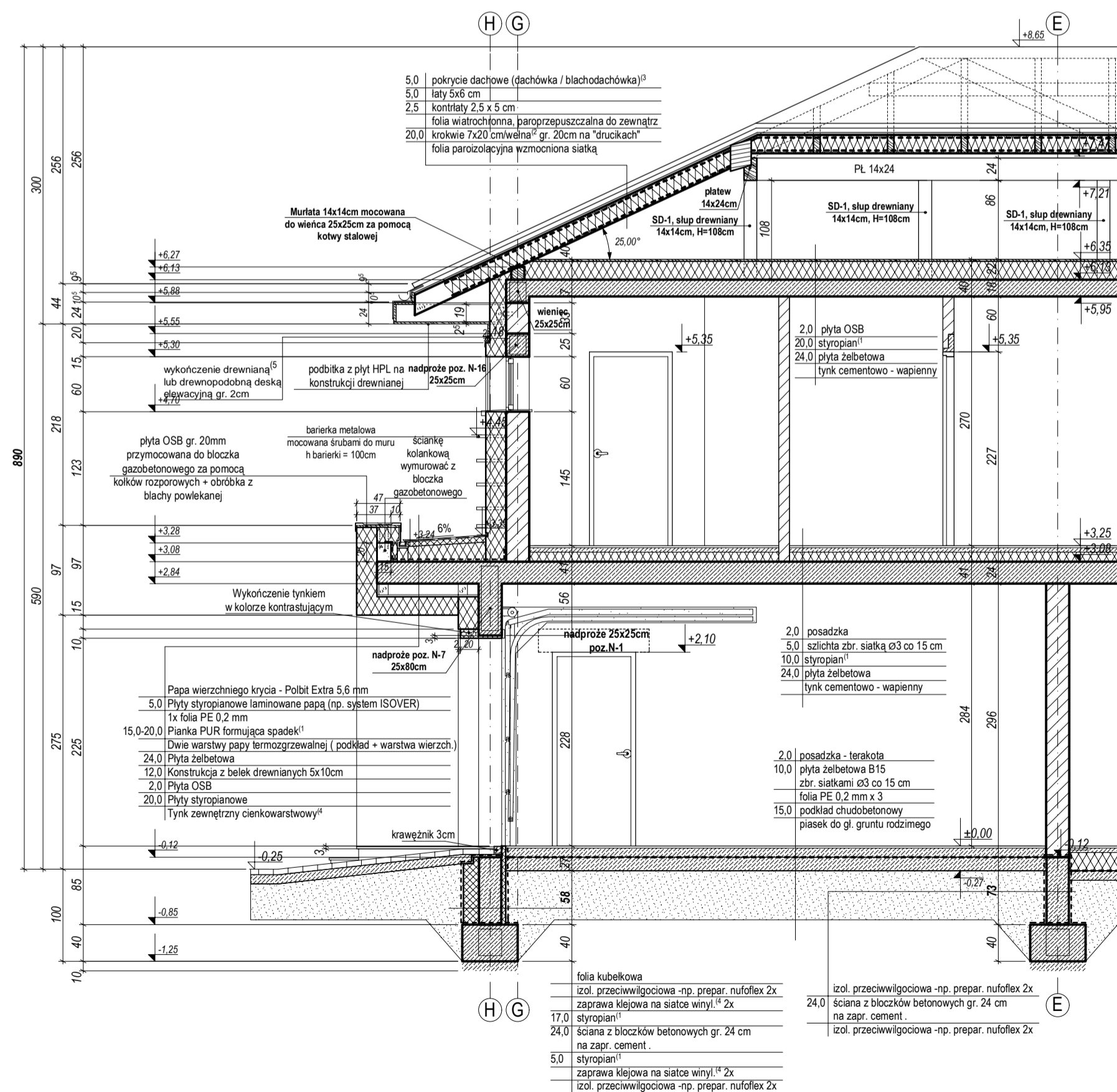
PRZEKRÓJ C - C
