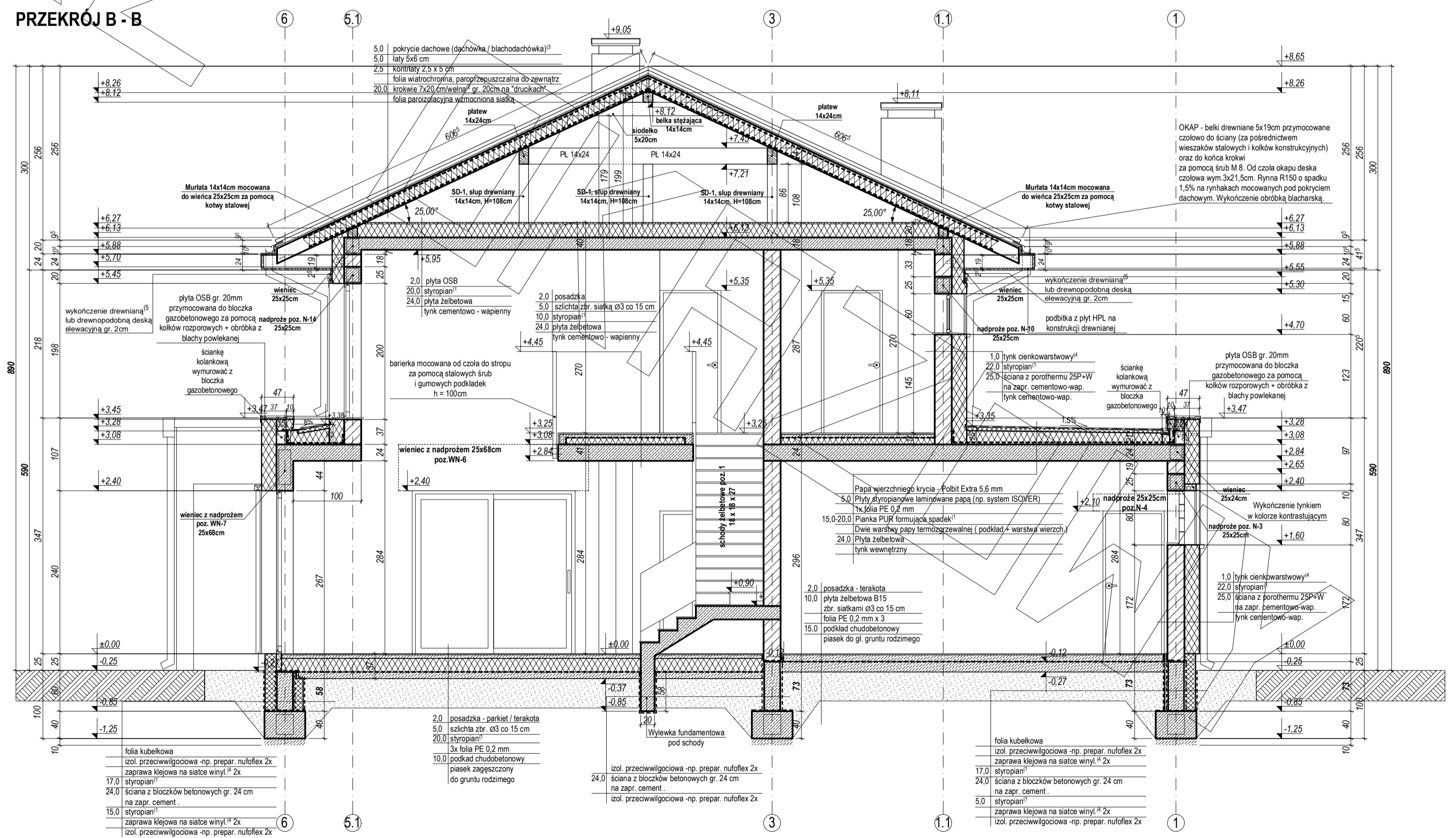
PRZEKRÓJ B - B
