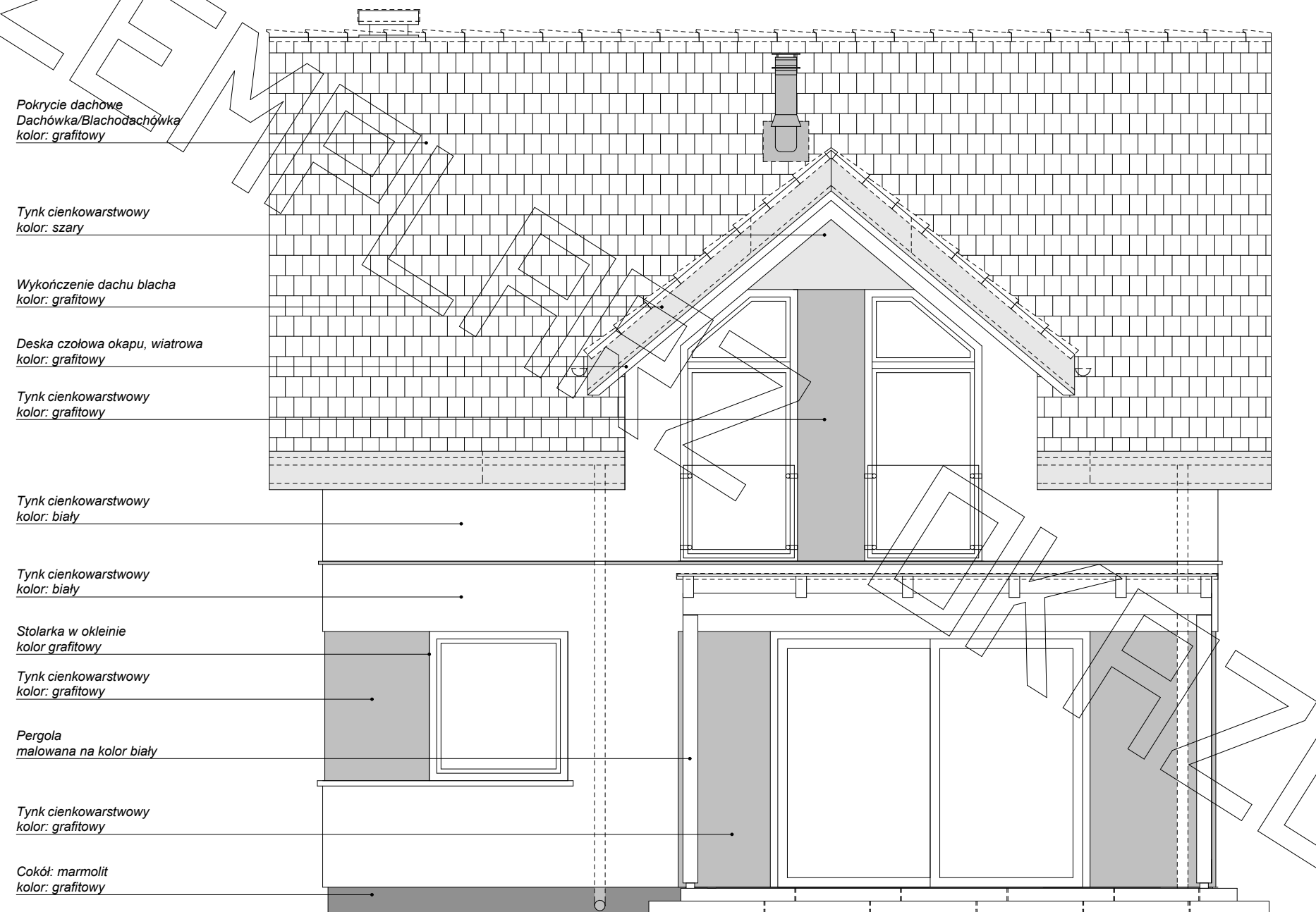
ELEWACJA TYLNA
