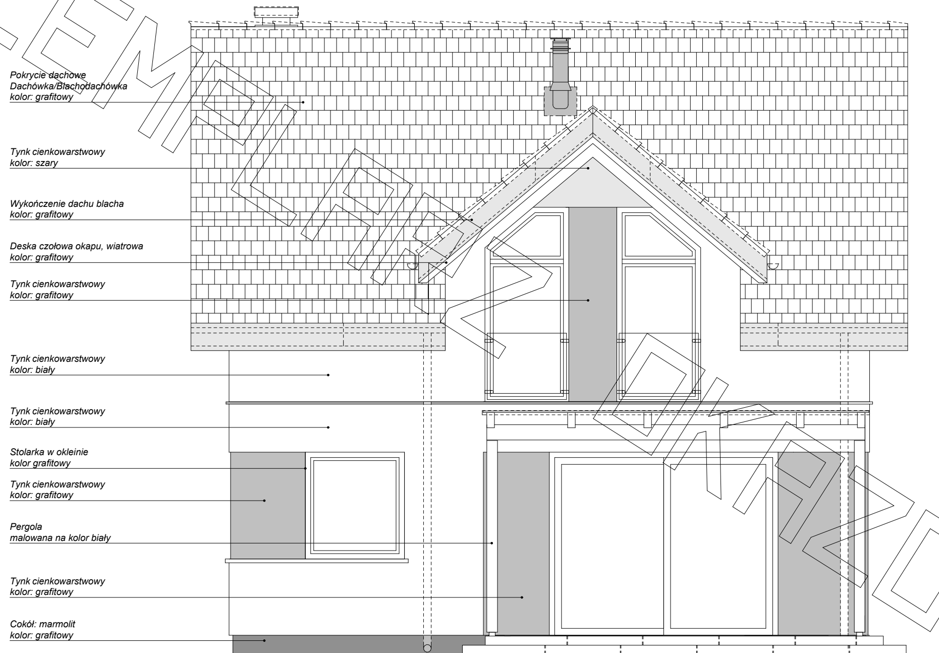
ELEWACJA TYLNA
