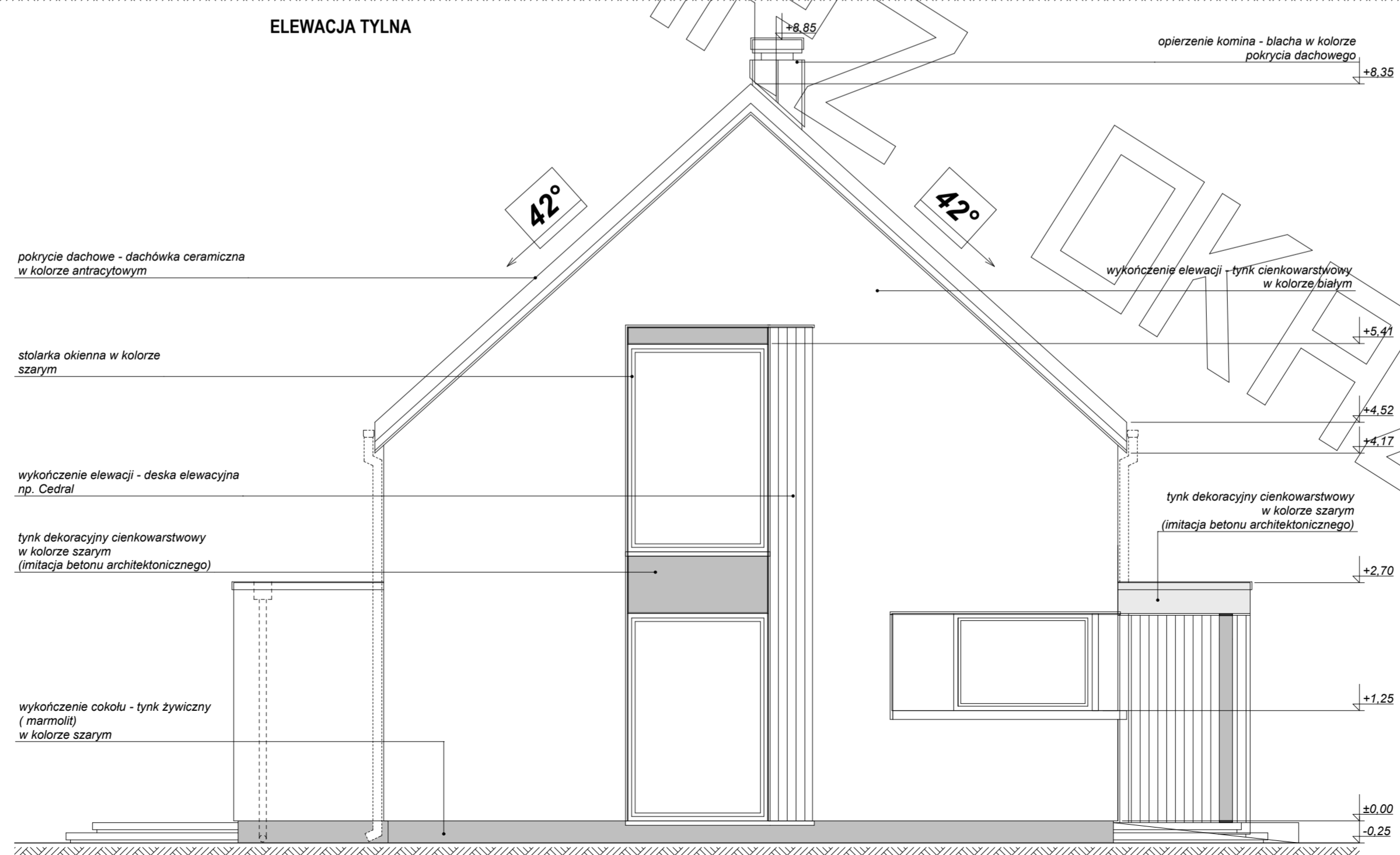
ELEWACJA PRZEDZIA
