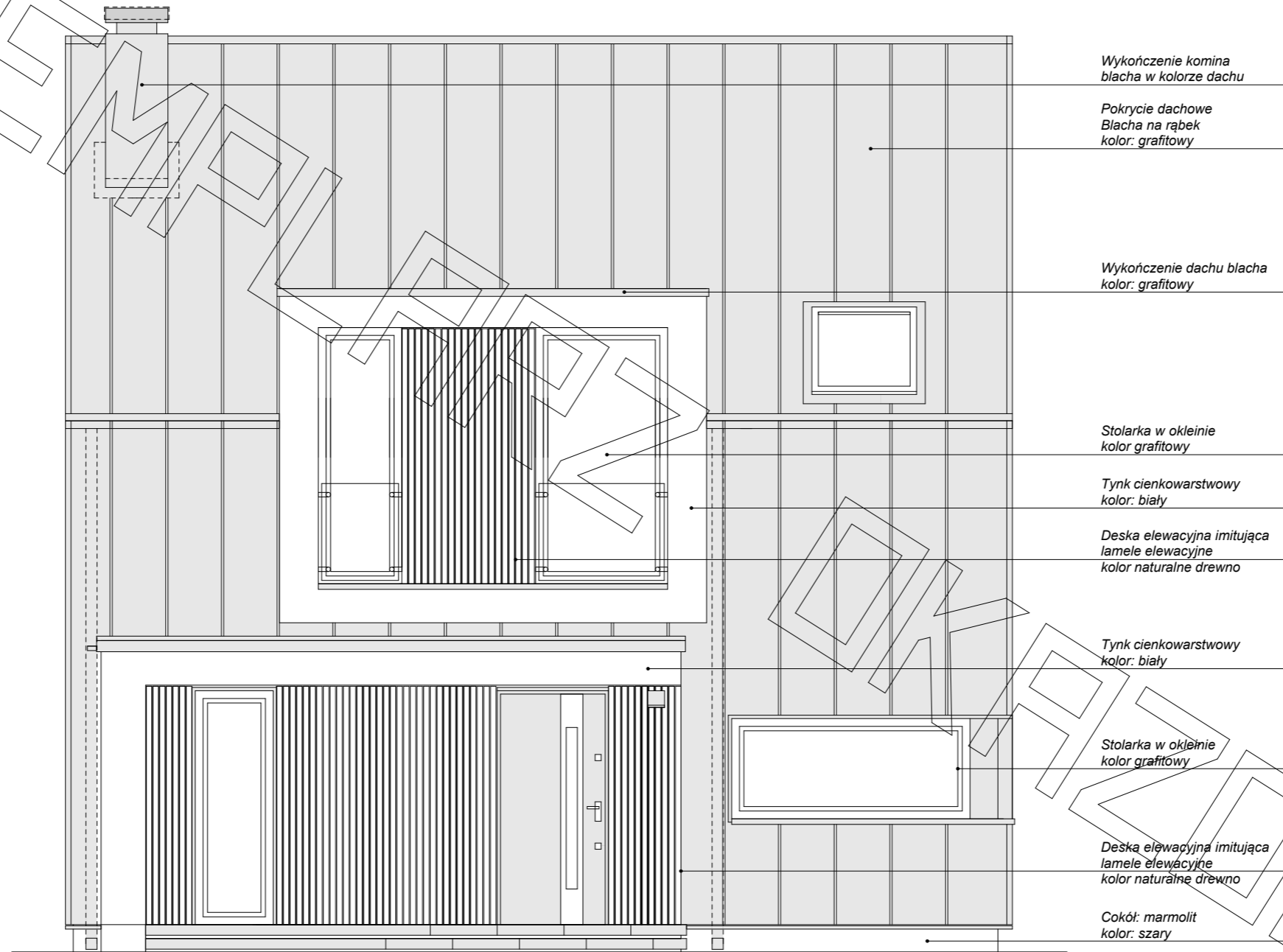
ELEWACJA FRONTOWA
