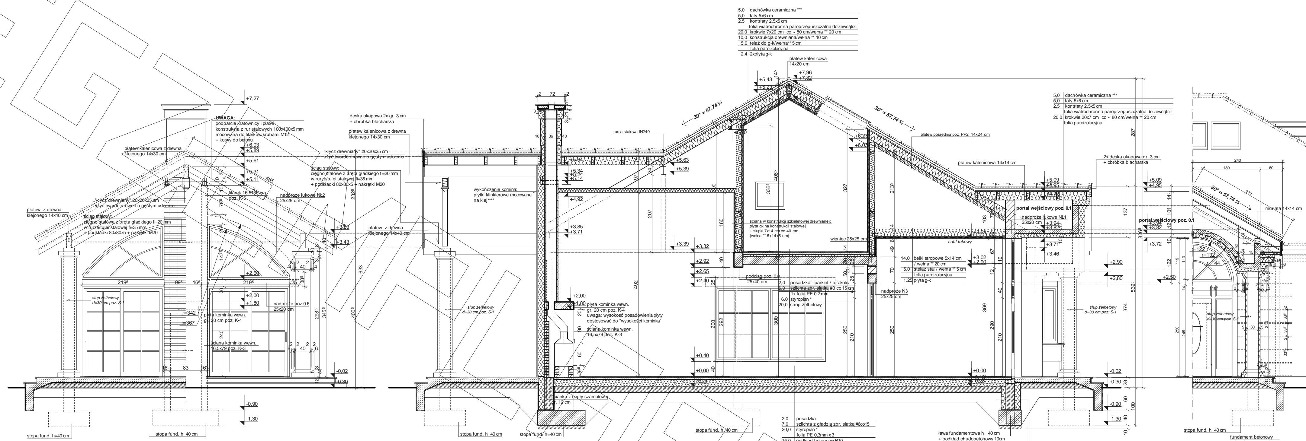
PRZEKRÓJ A-A
