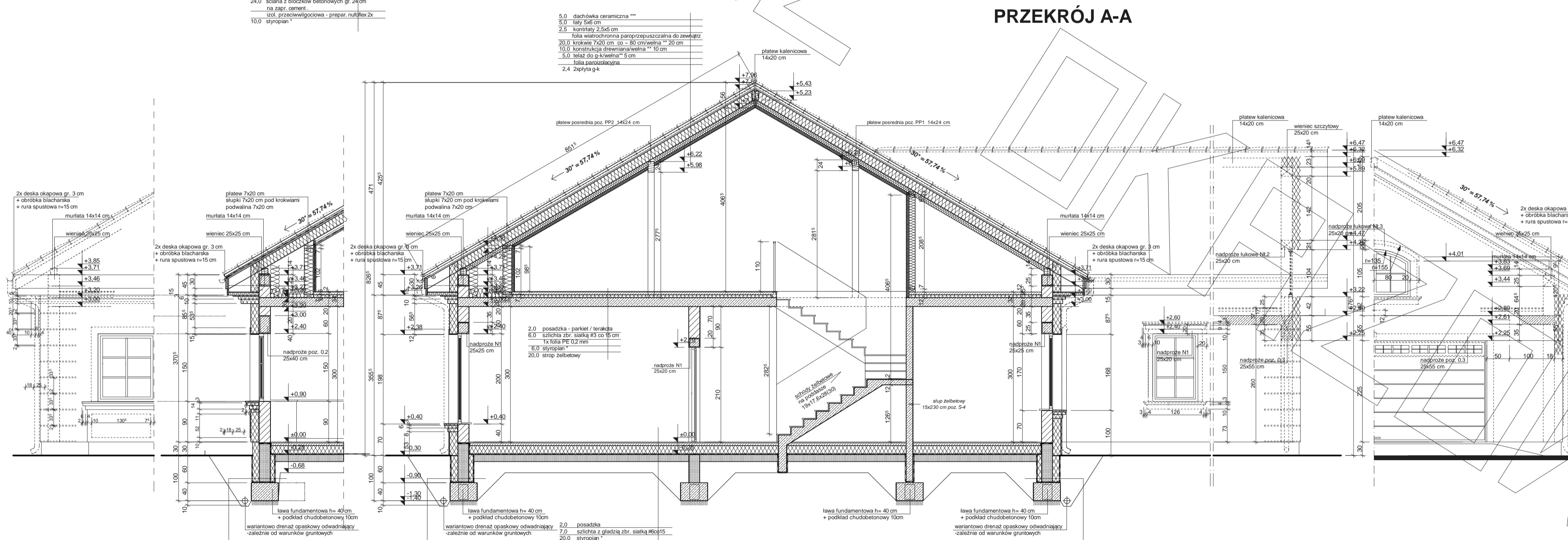
PRZEKRÓJ C
