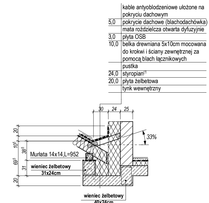
Detal odwodnienia dachu przekrój A1
