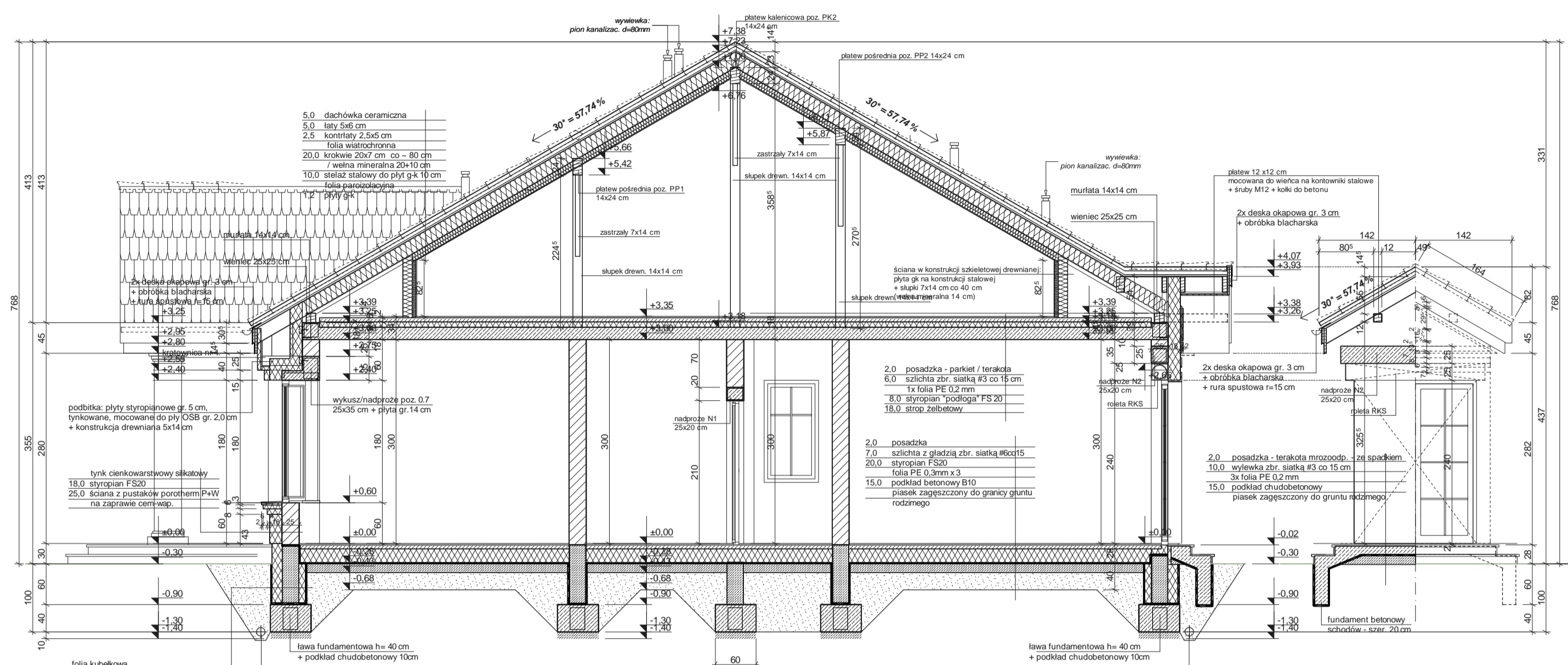
PRZEKRÓJ A-A
