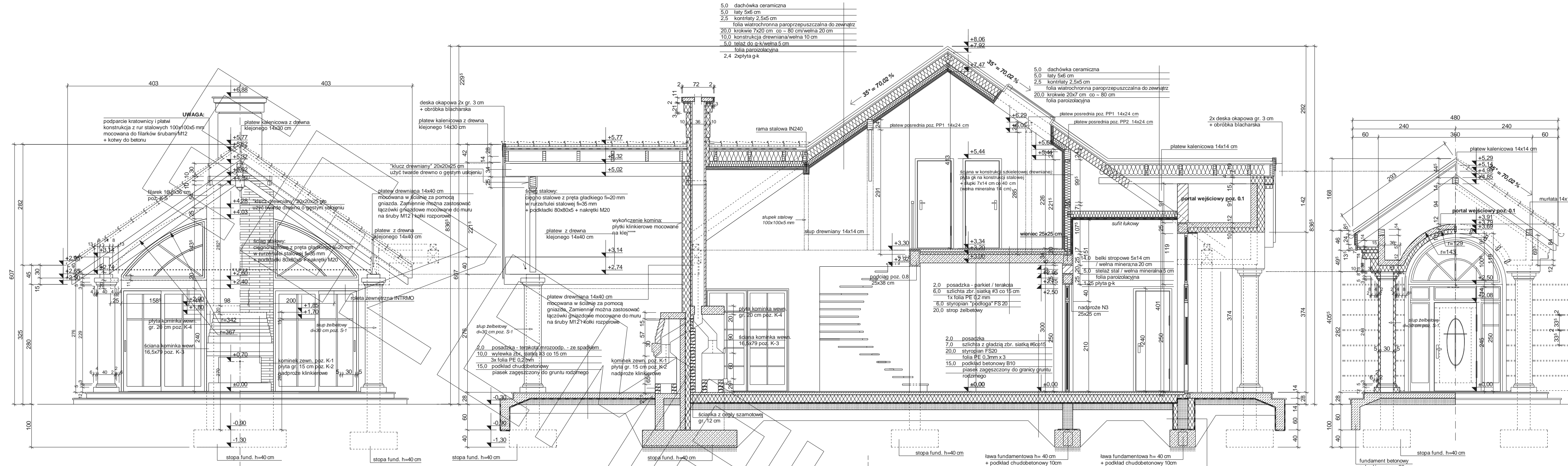
PRZEKRÓJ A-A
