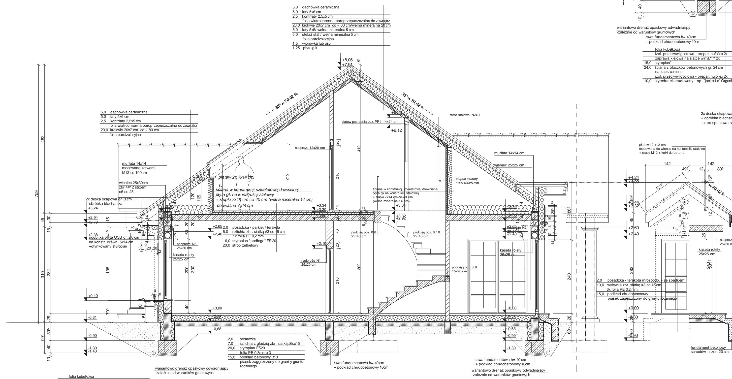
PRZEKRÓJ B-B
