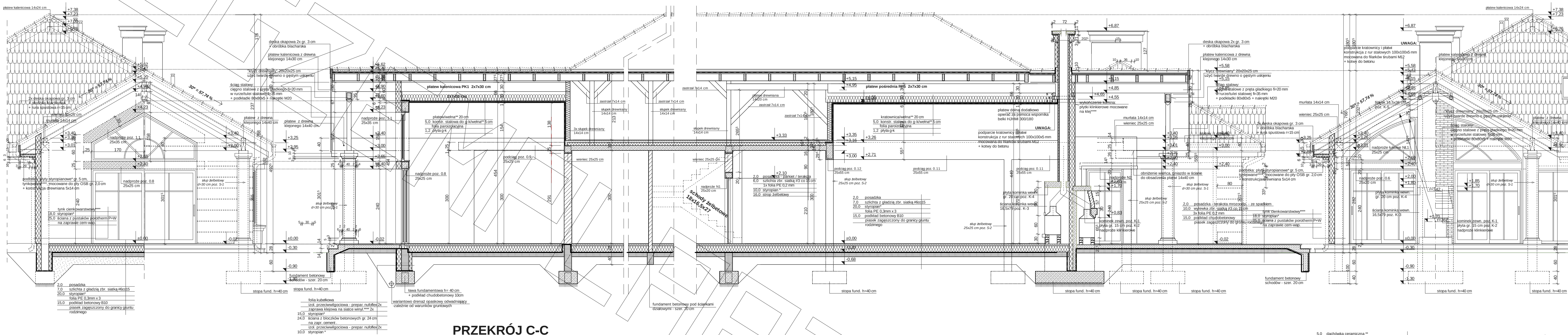
PRZEKRÓJ C-C
