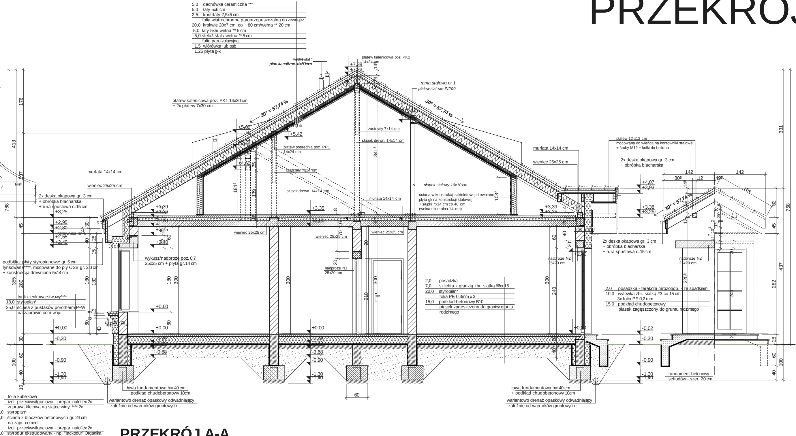
PRZEKRÓJ A-A
