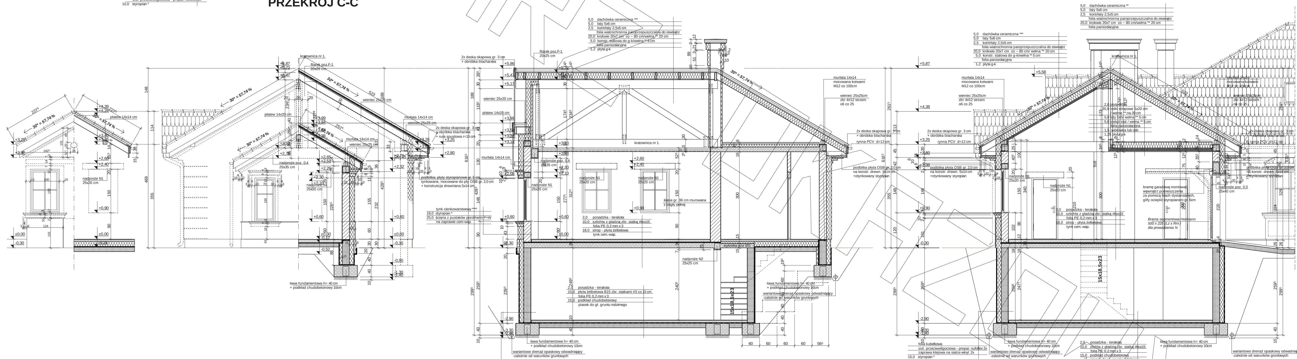
PRZEKRÓJ E
