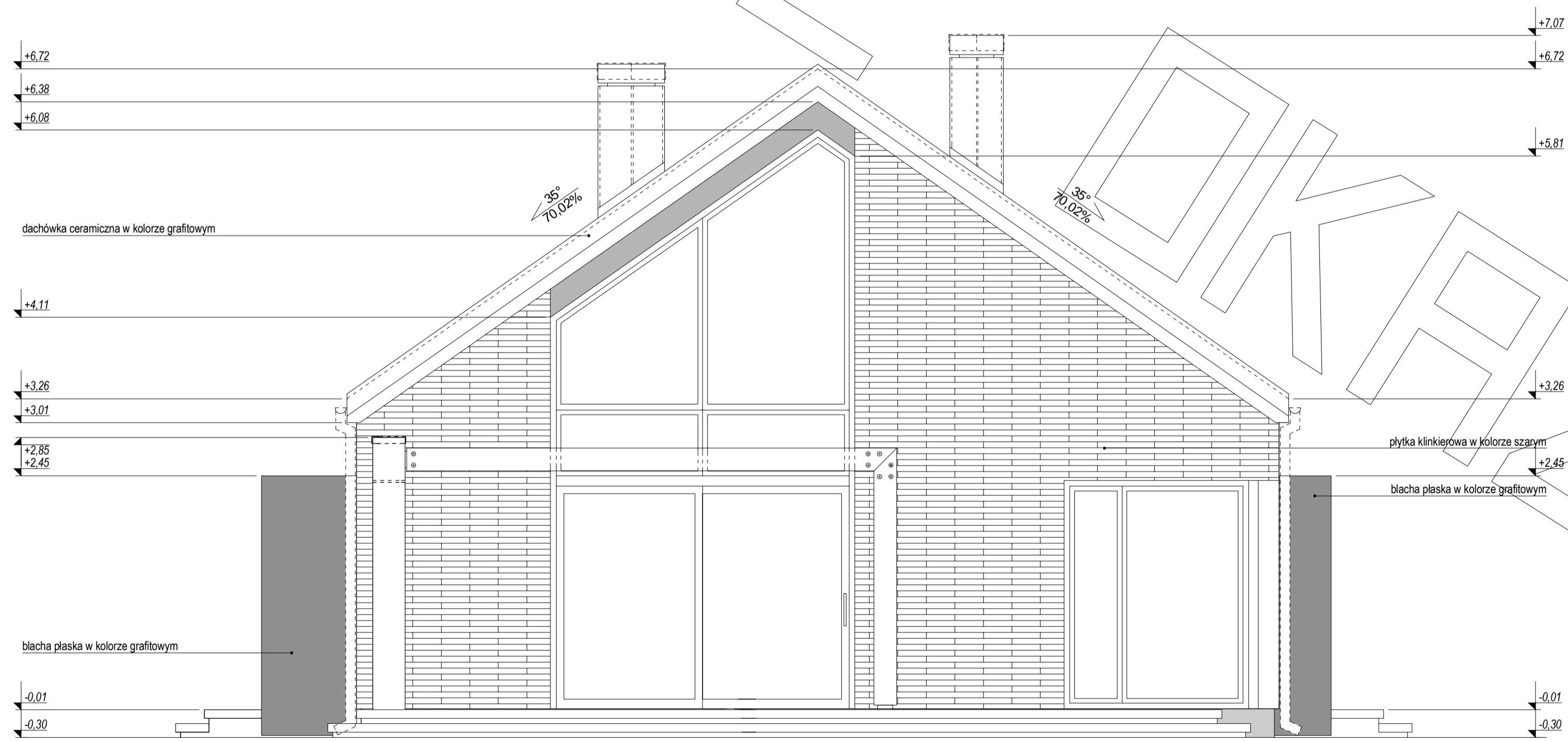
ELEWACJA BOCZNA:
