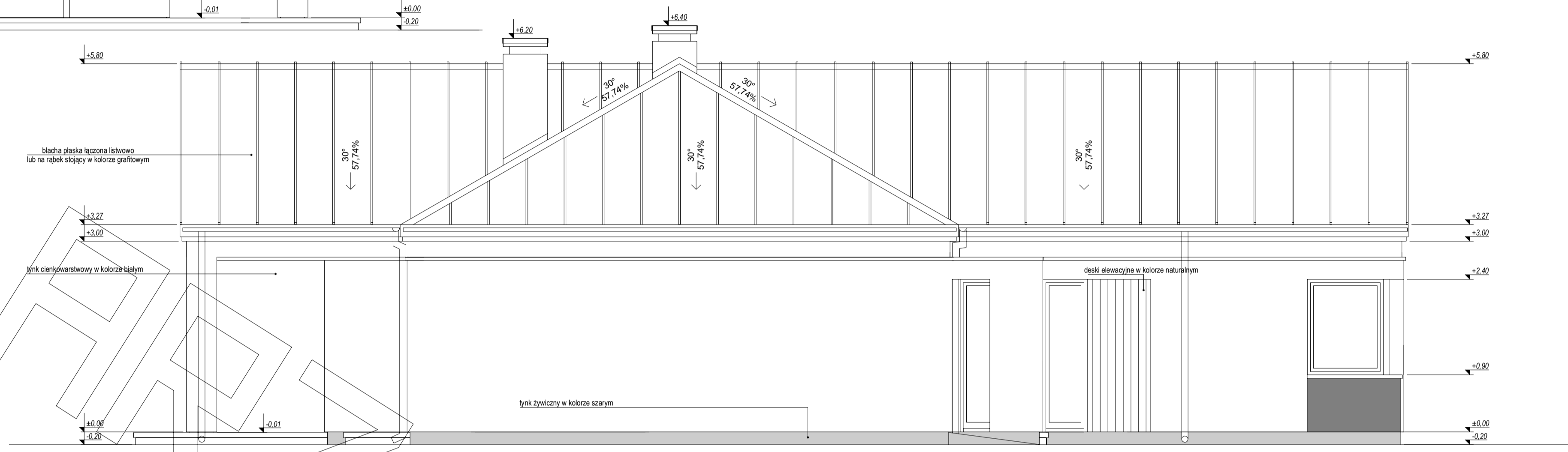
ELEWACJA BOCZNA:
