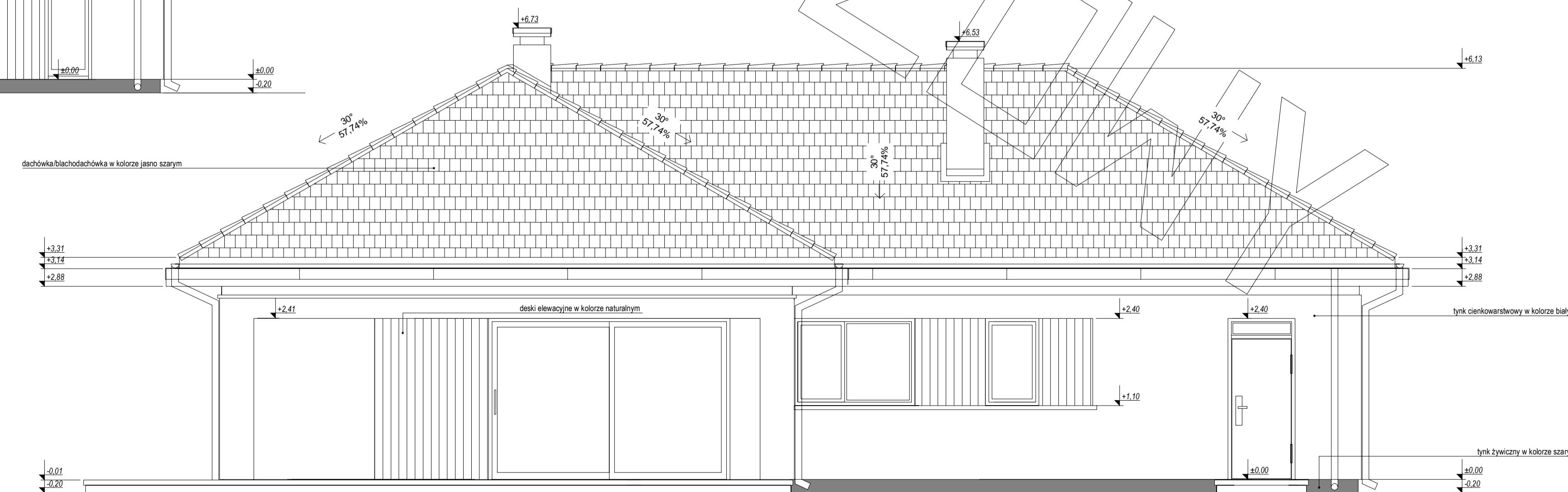
ELEWACJA TYLNA:
