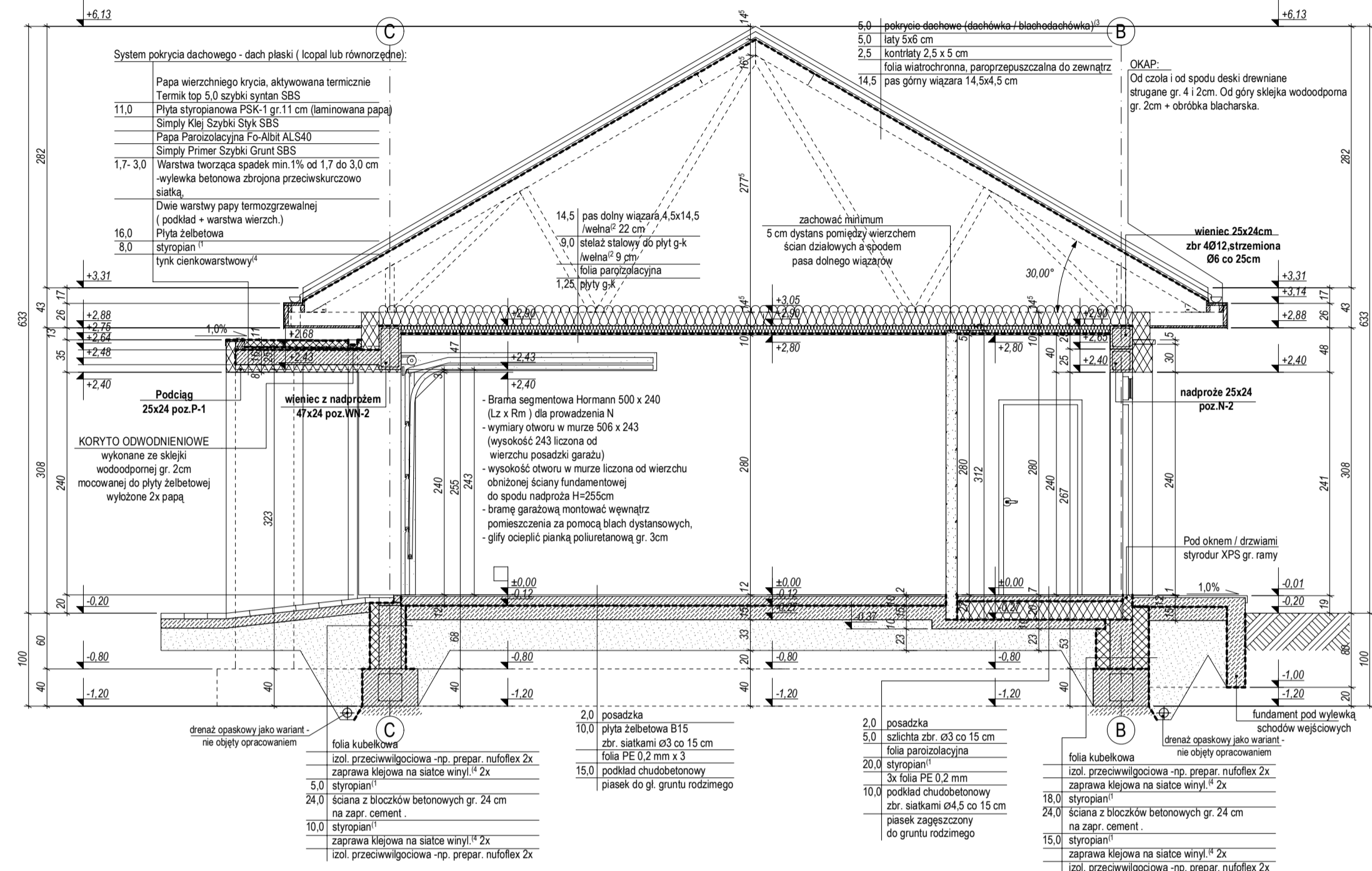
PRZEKRÓJ B1 - B1
