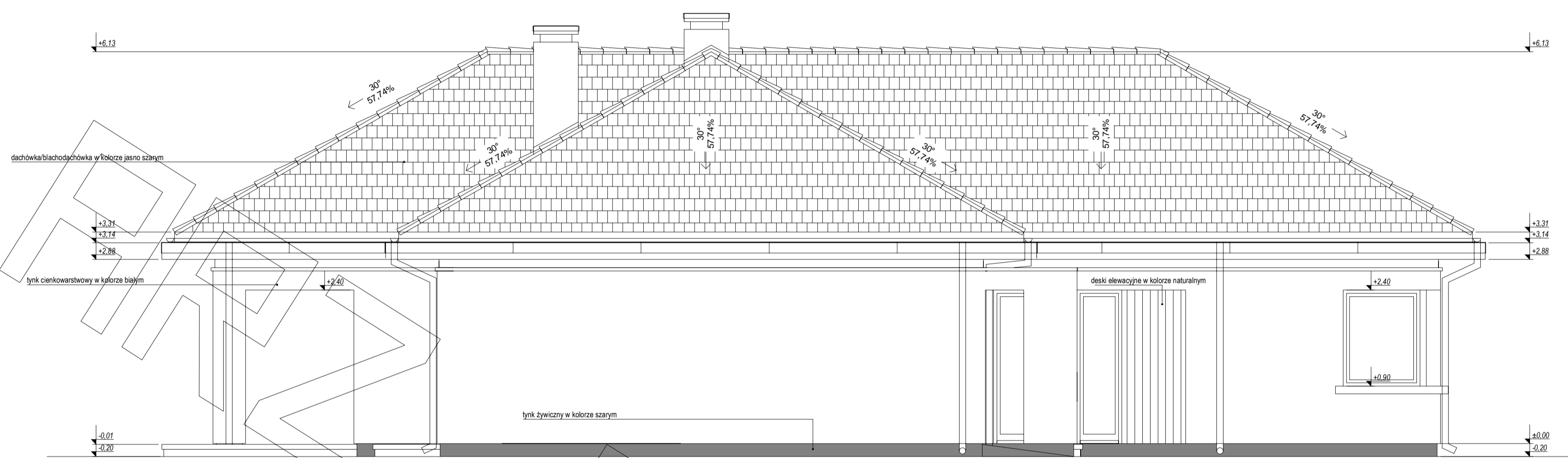
ELEWACJA BOCZNA:
