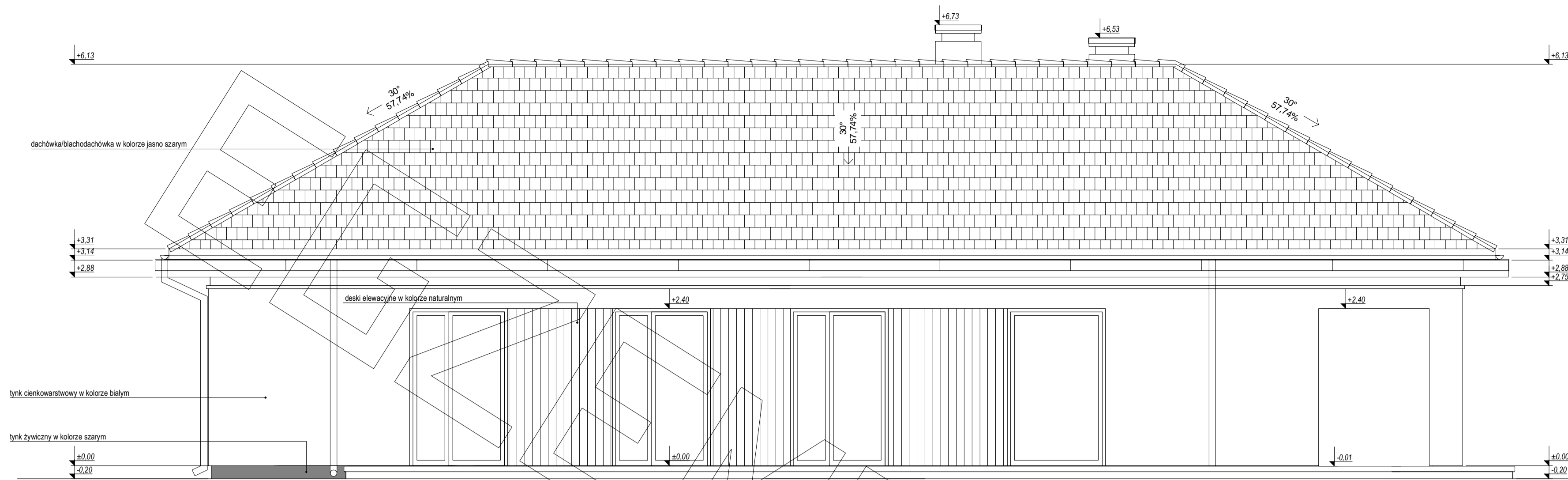
ELEWACJA BOCZNA:
