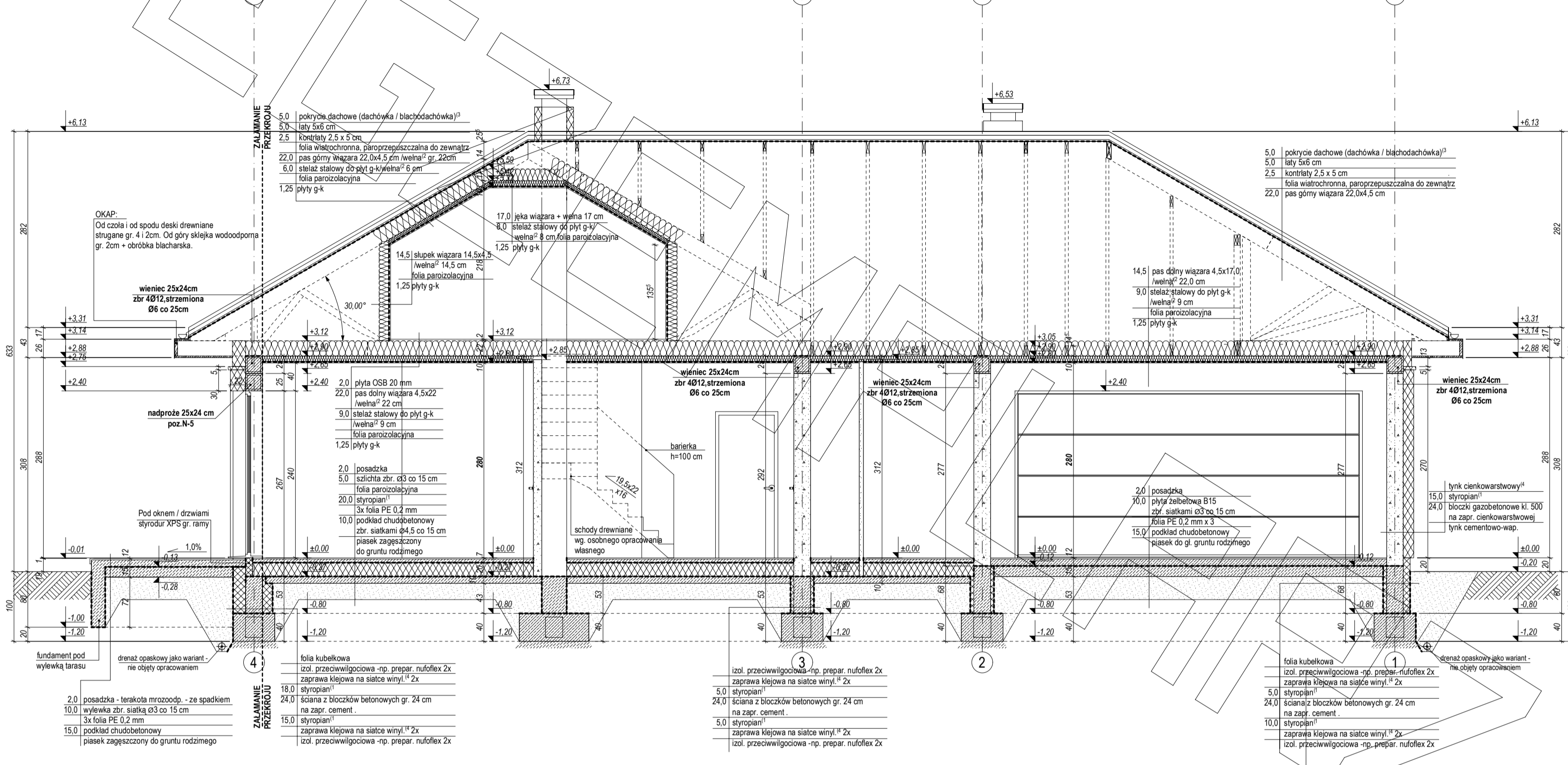
PRZEKRÓJ B - B
