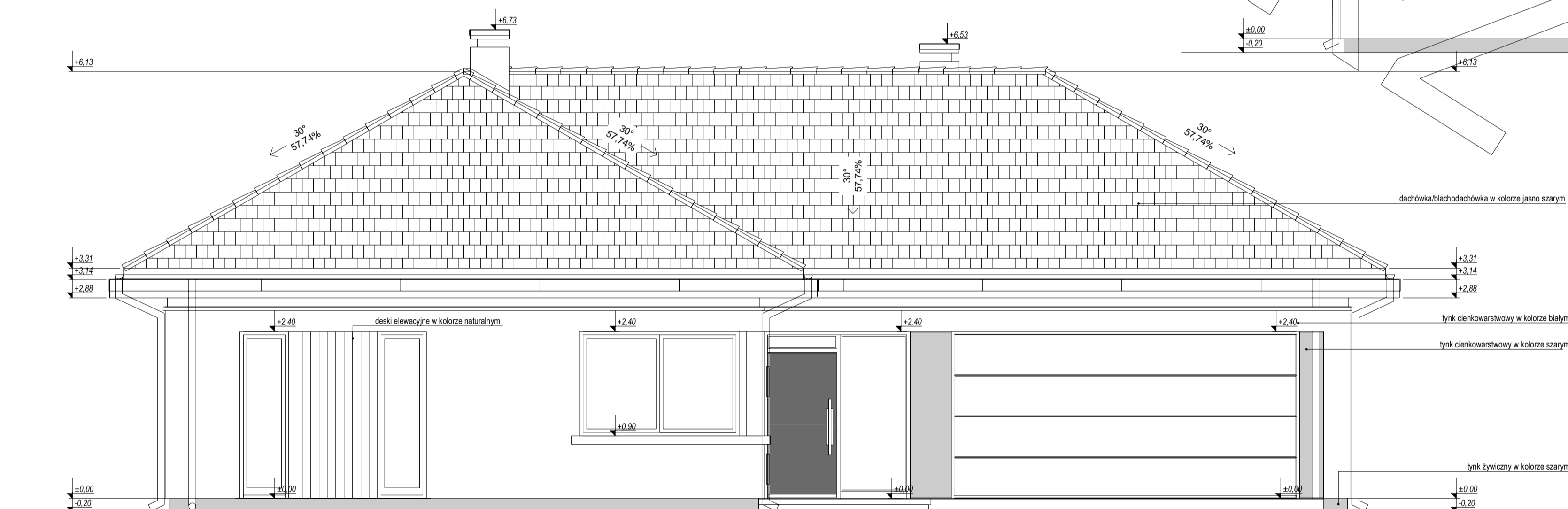
ELEWACJA FRONTOWA:
