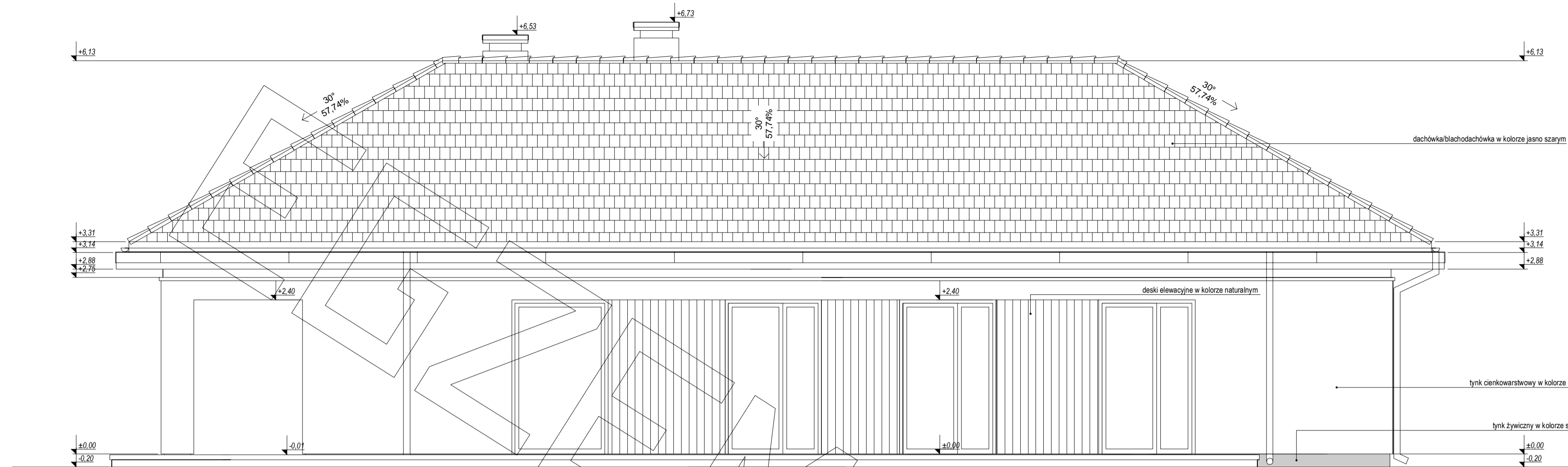
ELEWACJA BOCZNA:
