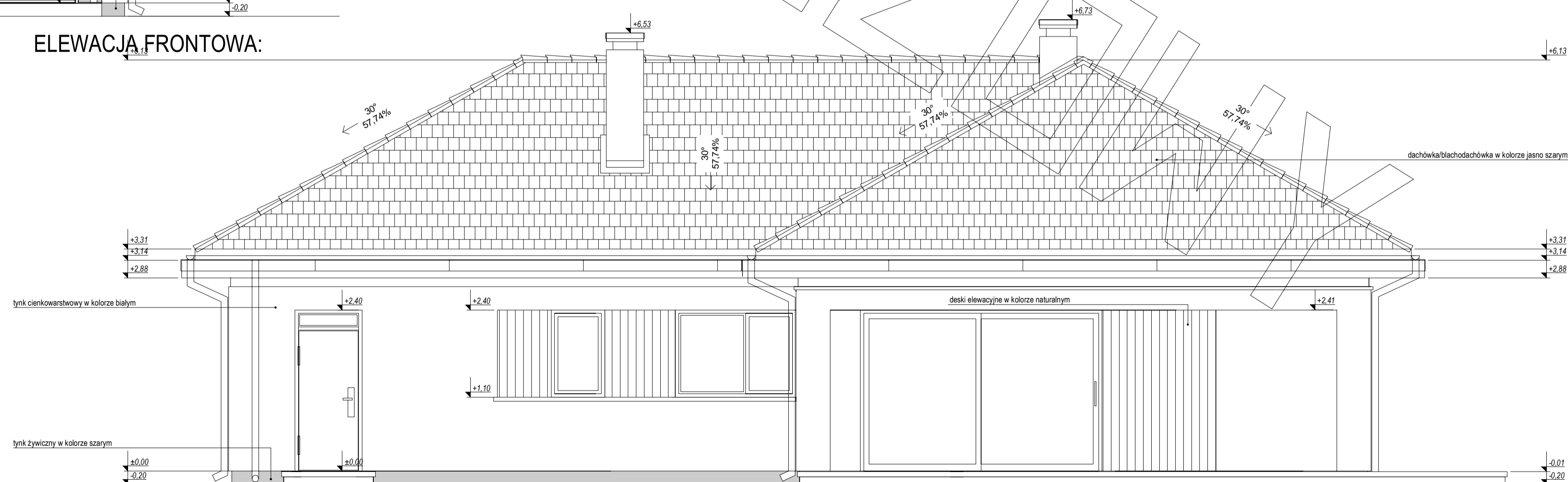
ELEWACJA TYLNA:
