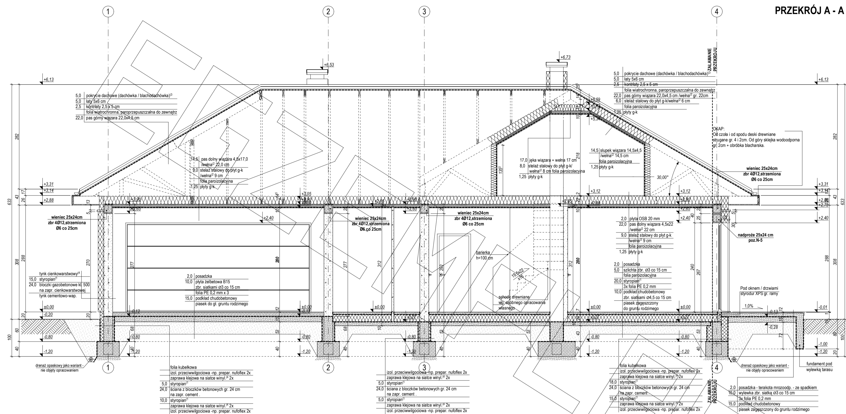
PRZEKRÓJ A - A
