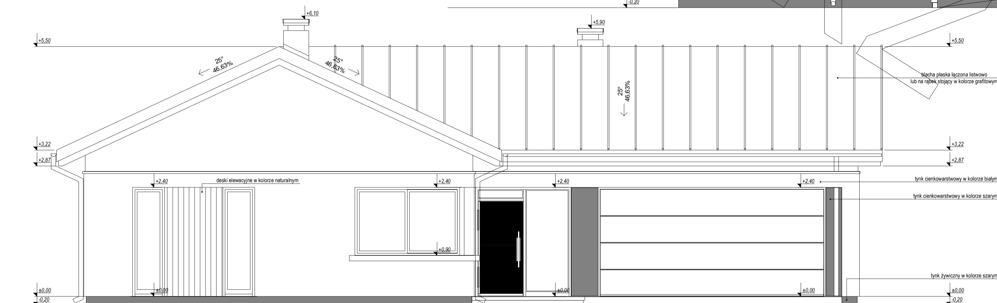
ELEWACJA FRONTOWA:
