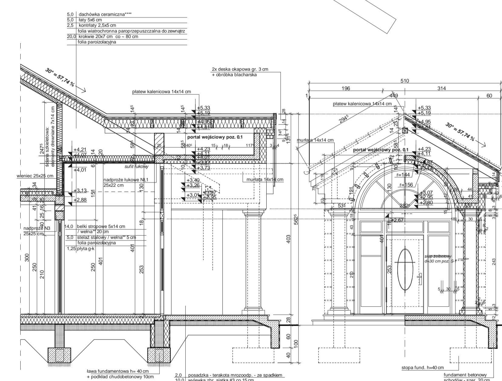
PRZEKRÓJ B'
