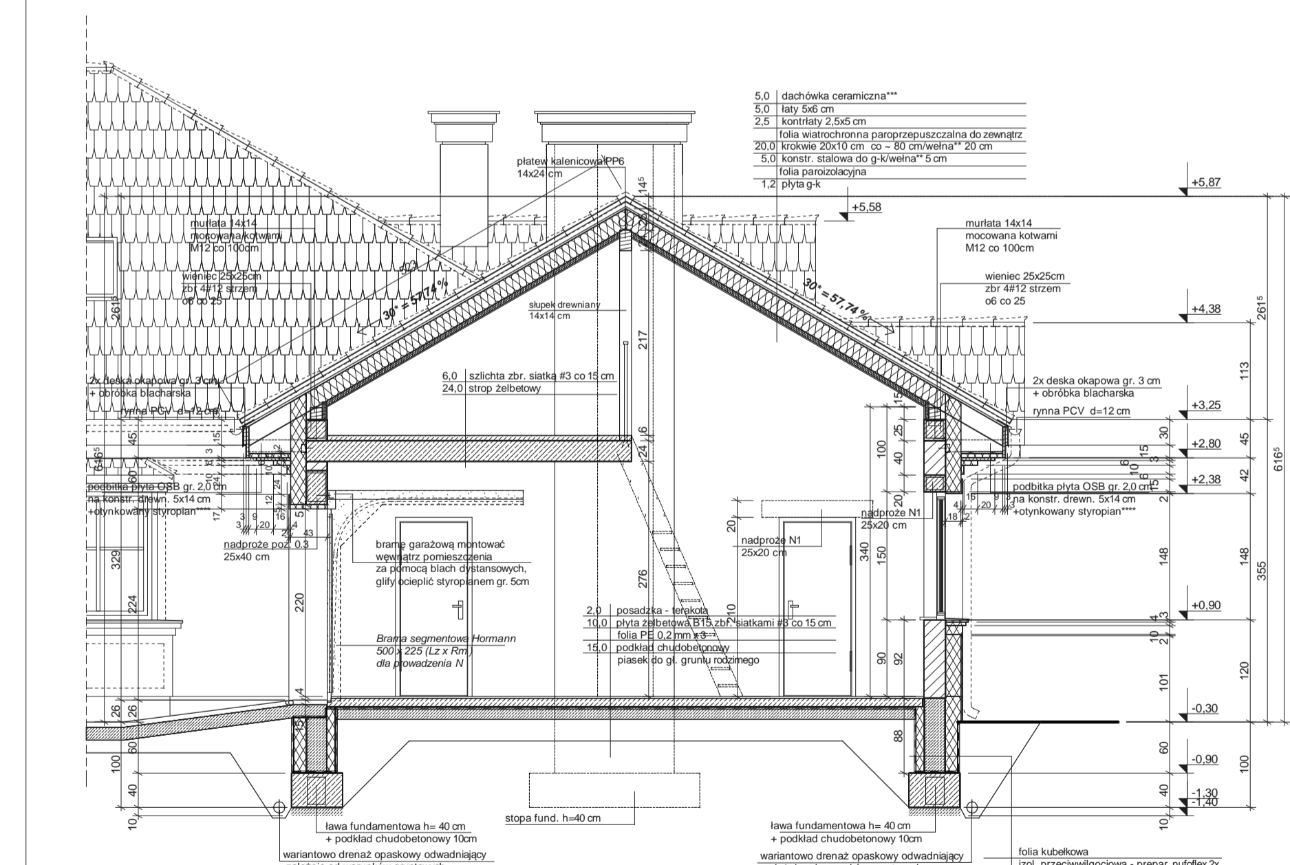
PRZEKRÓJ D-D
