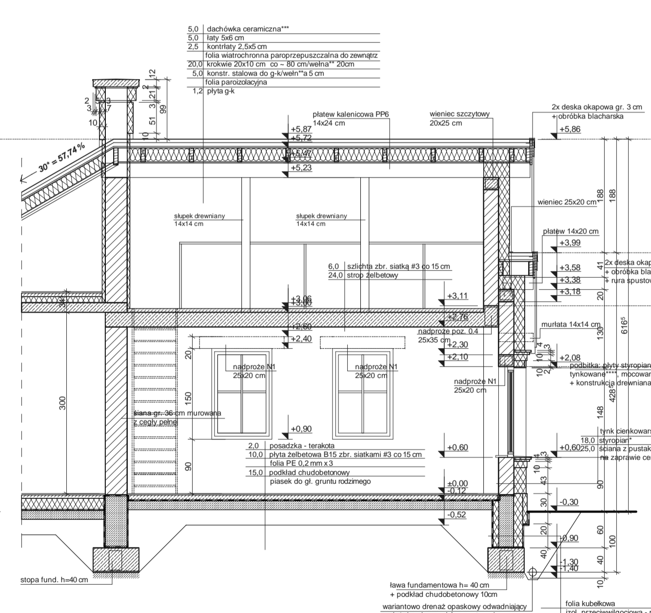
PRZEKRÓJ E
