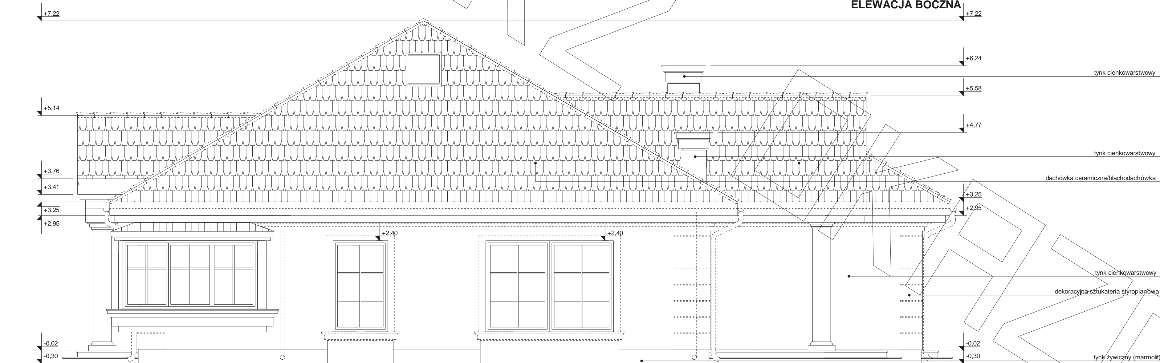
ELEWACJA BOCZNA
