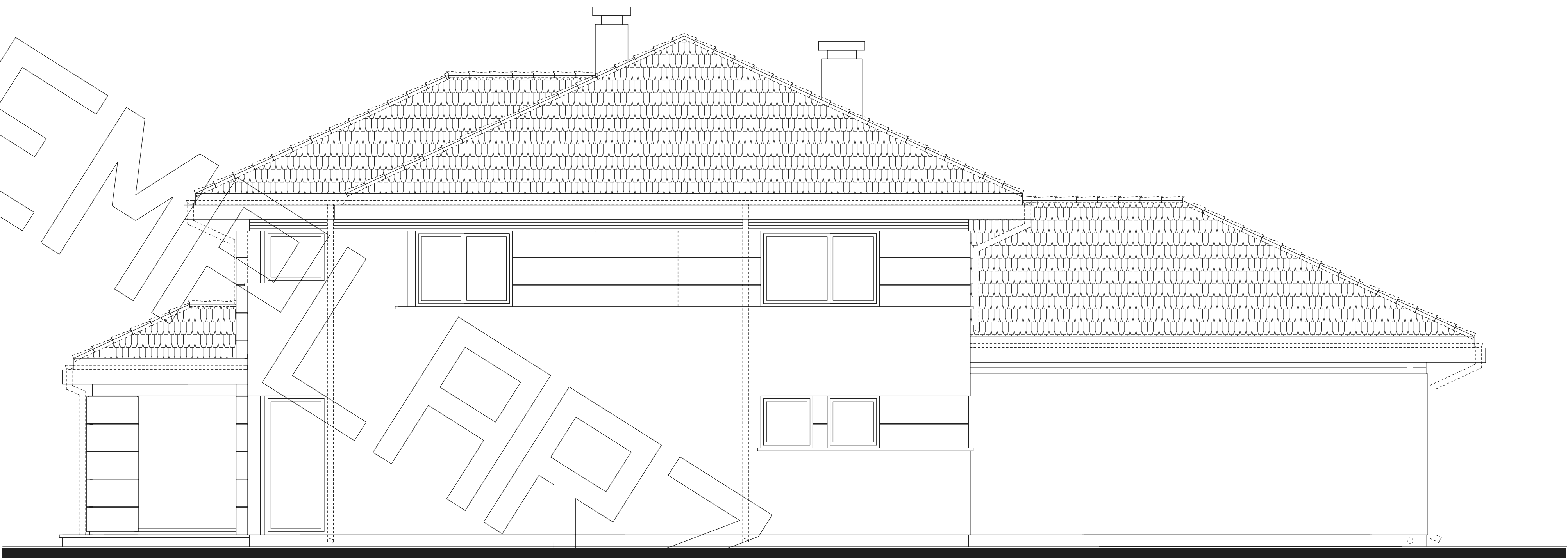
ELEWACJA TYLNA
