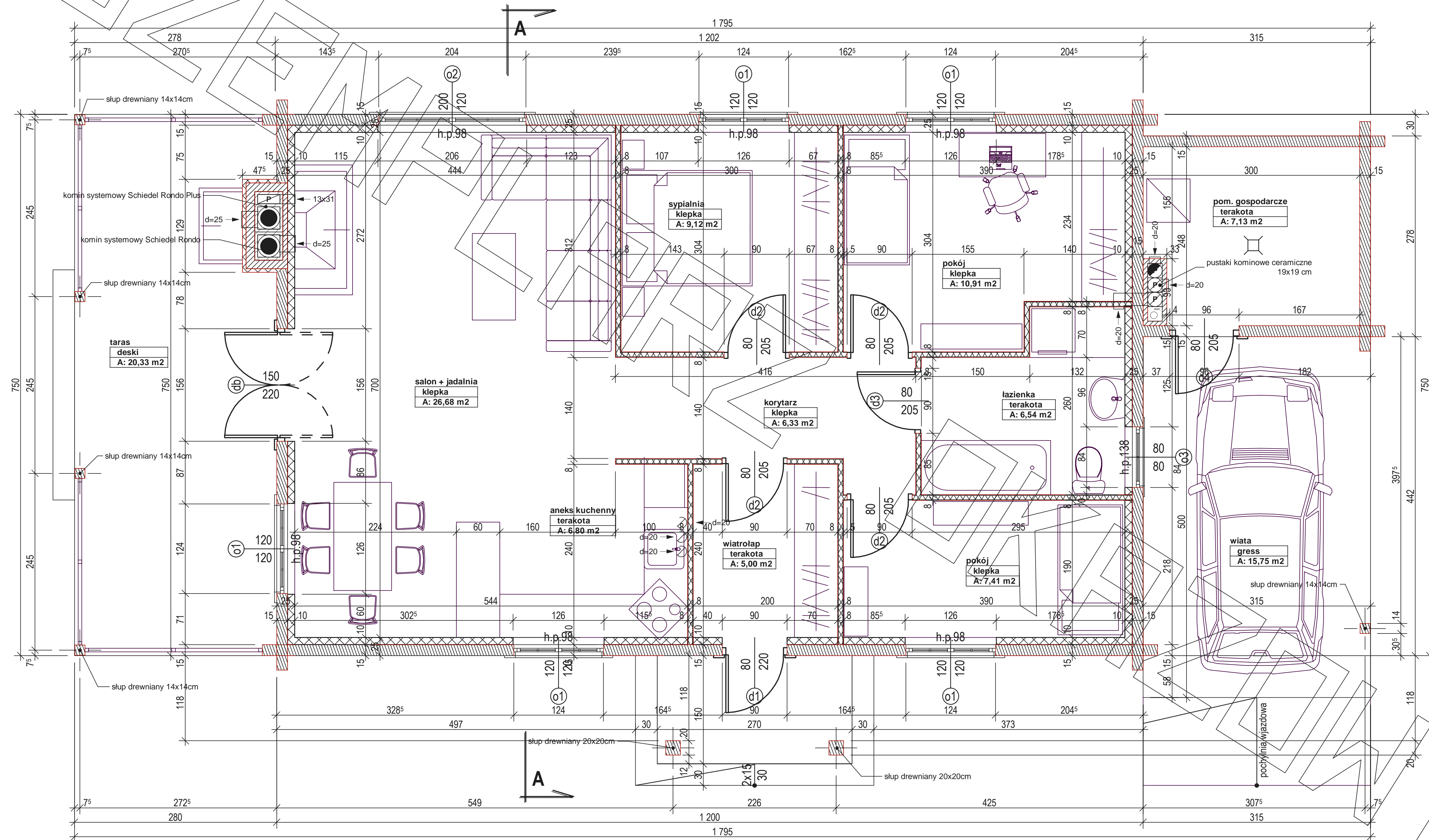
RZUT PARTERU
