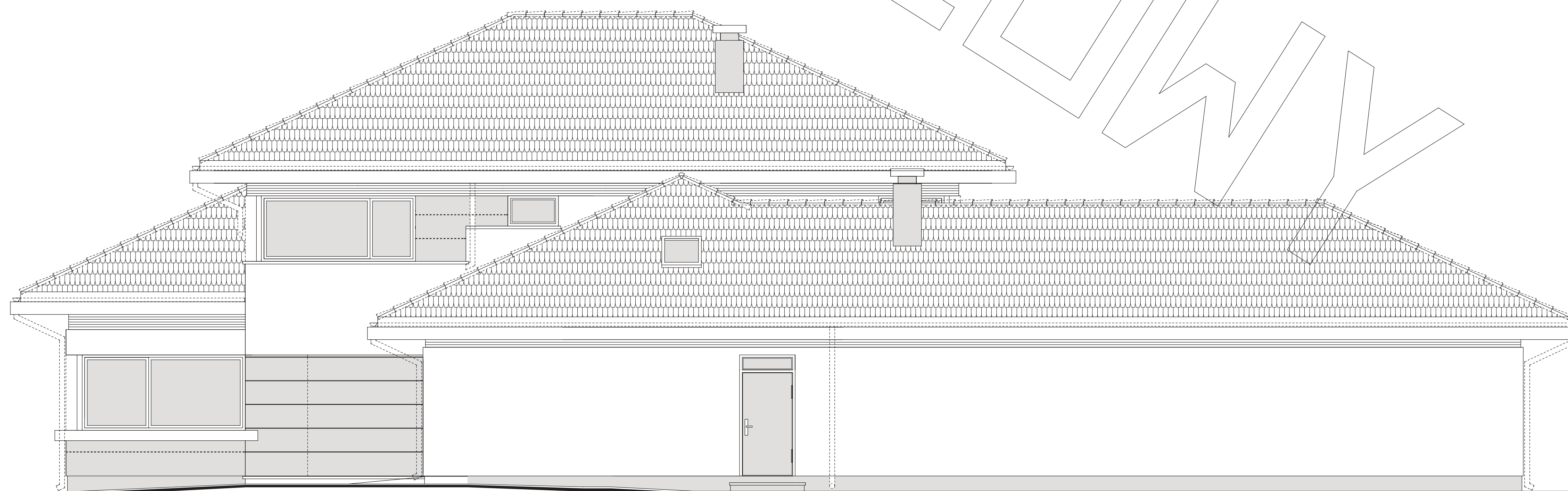
elewacja boczna
