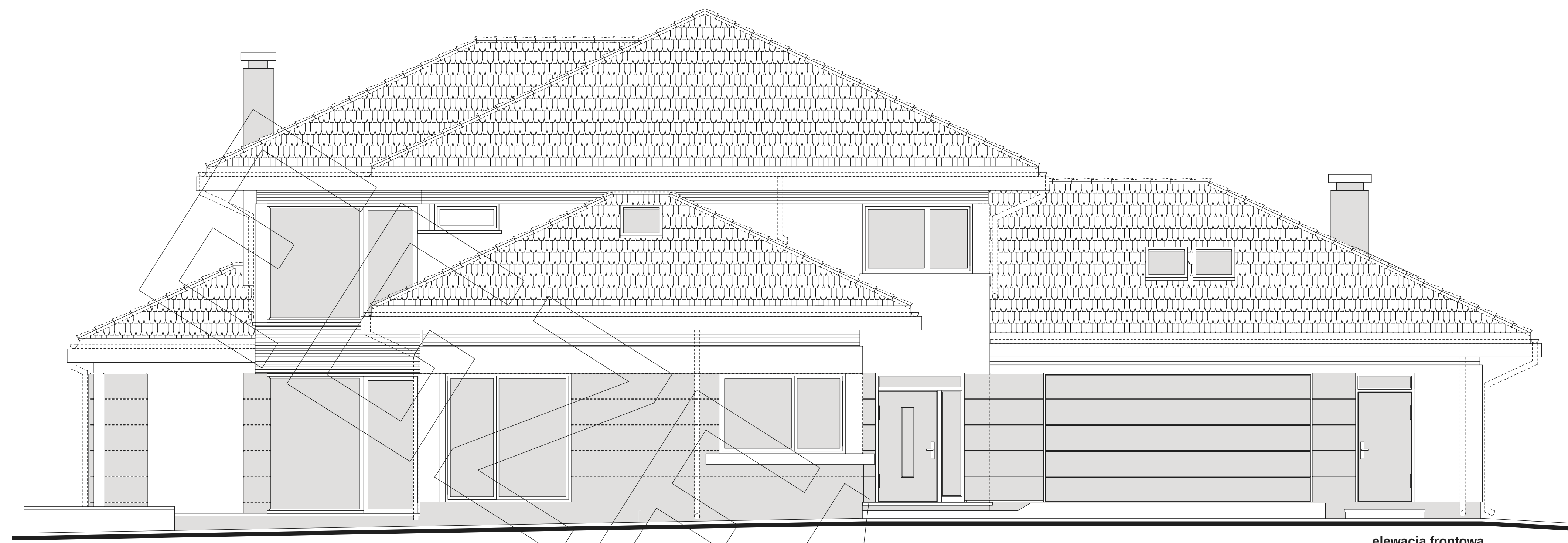
elewacja frontowa
