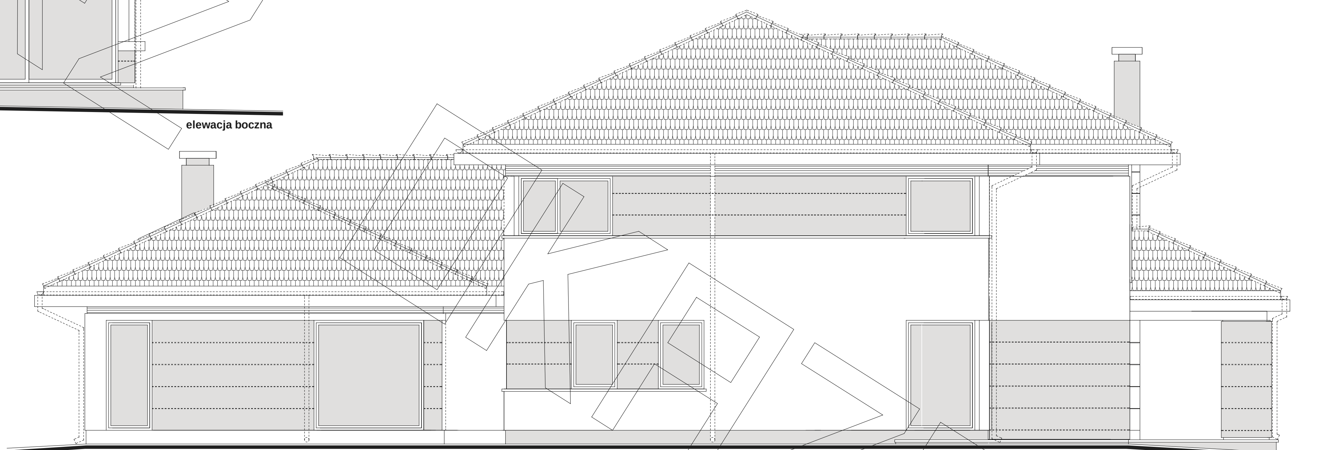
elewacja tylna
