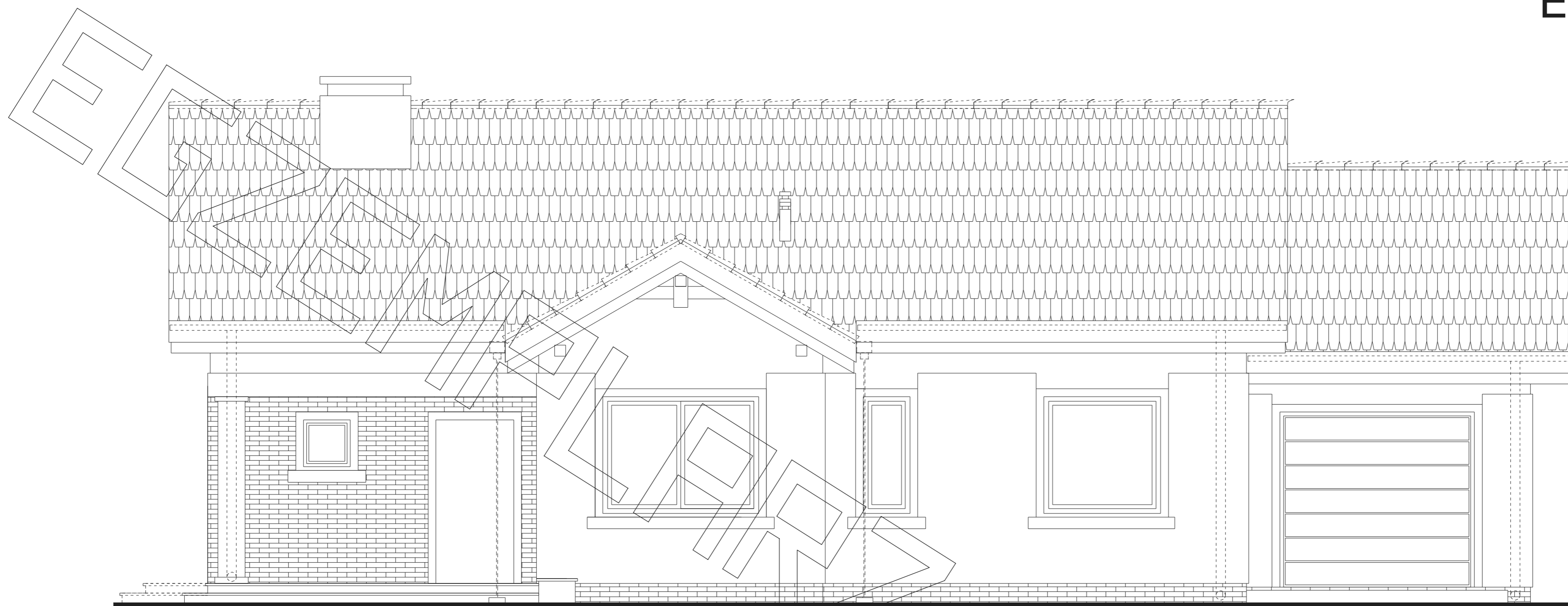
elewacja frontowa
