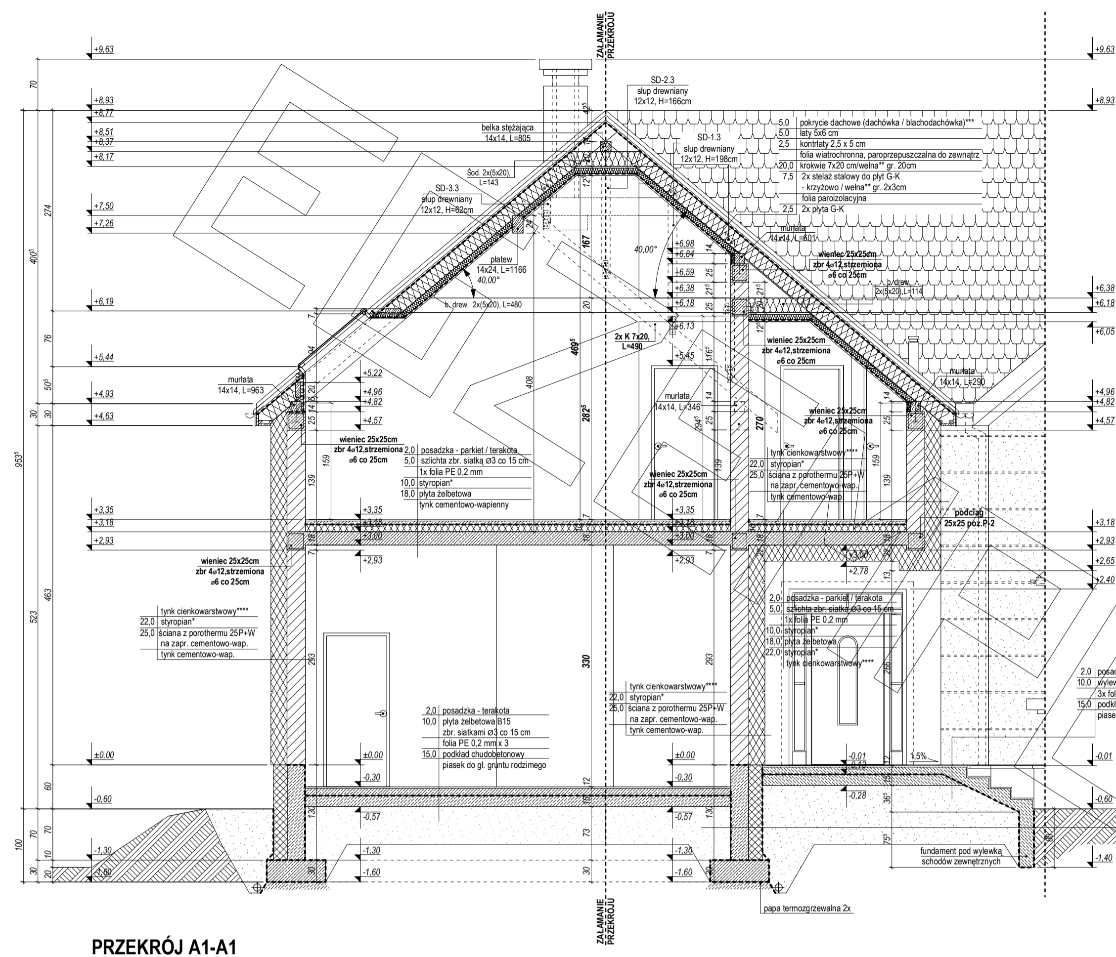
PRZEKRÓJ A1-A1
