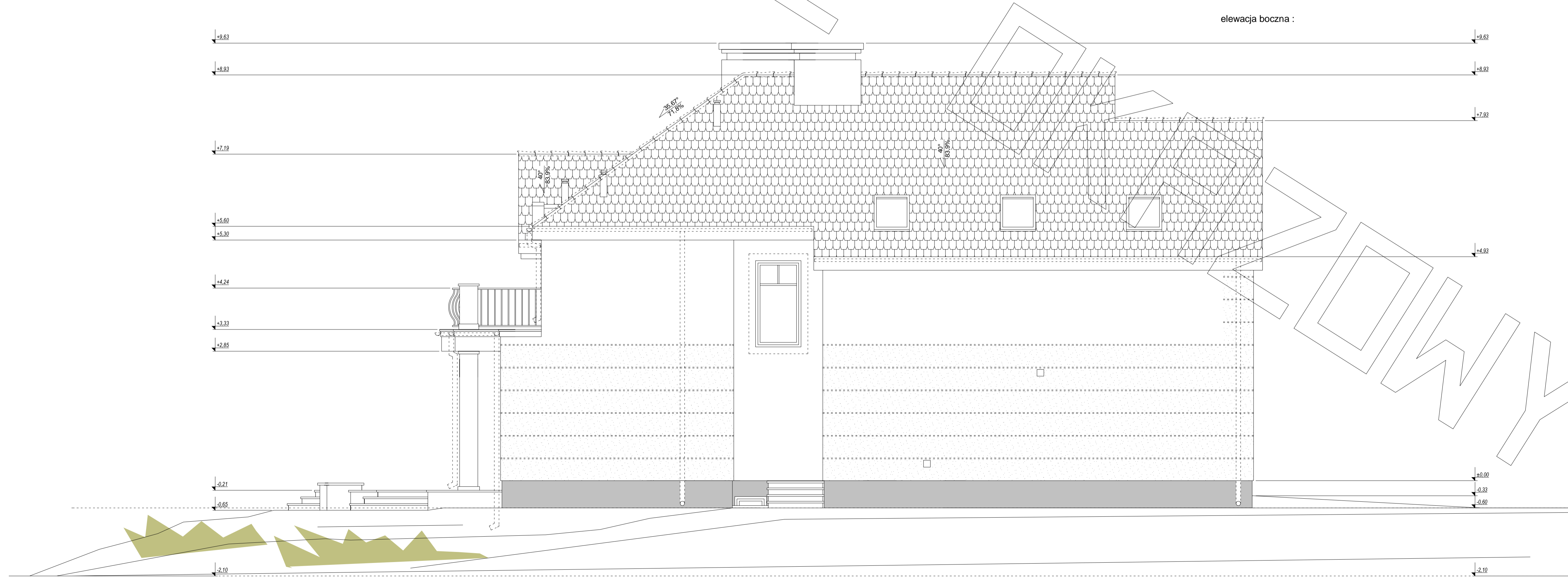
elewacja boczna :
