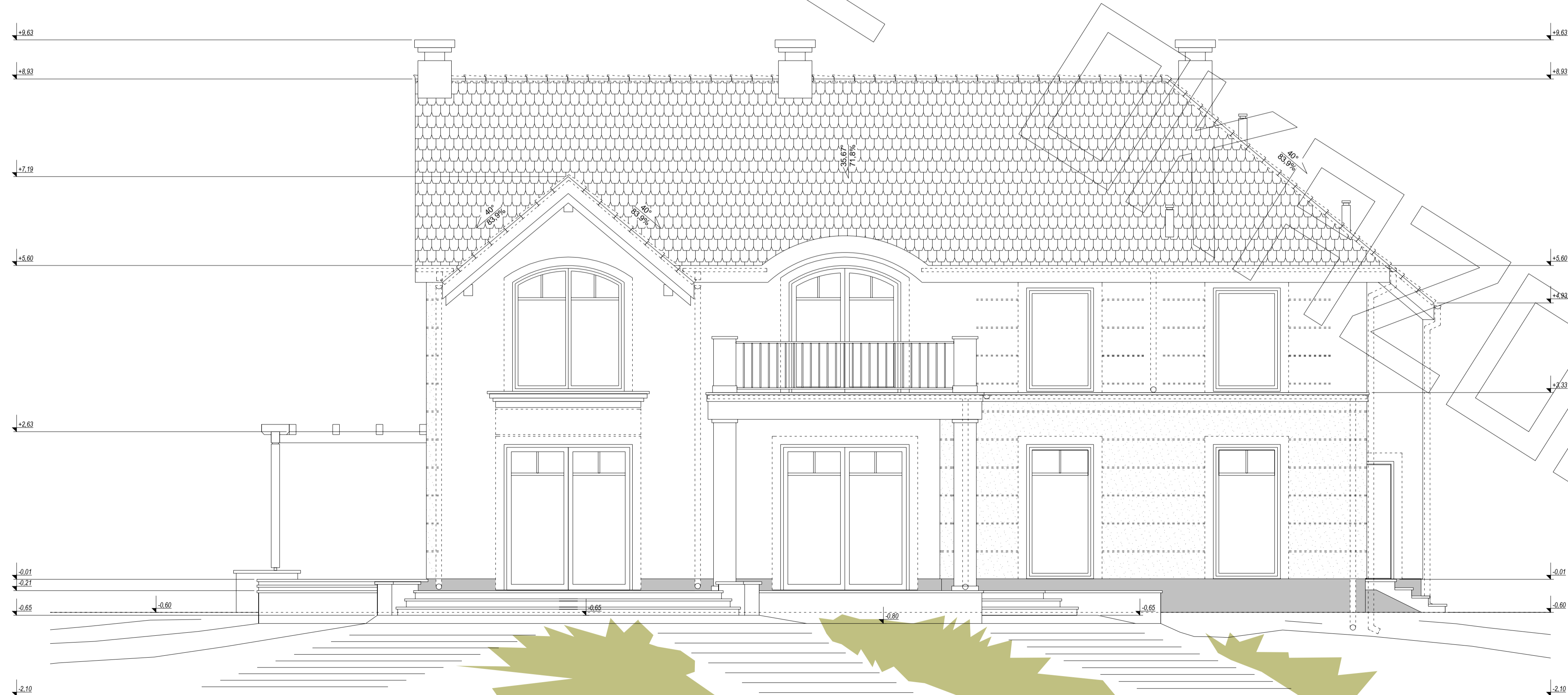
elewacja ogrodowa :
