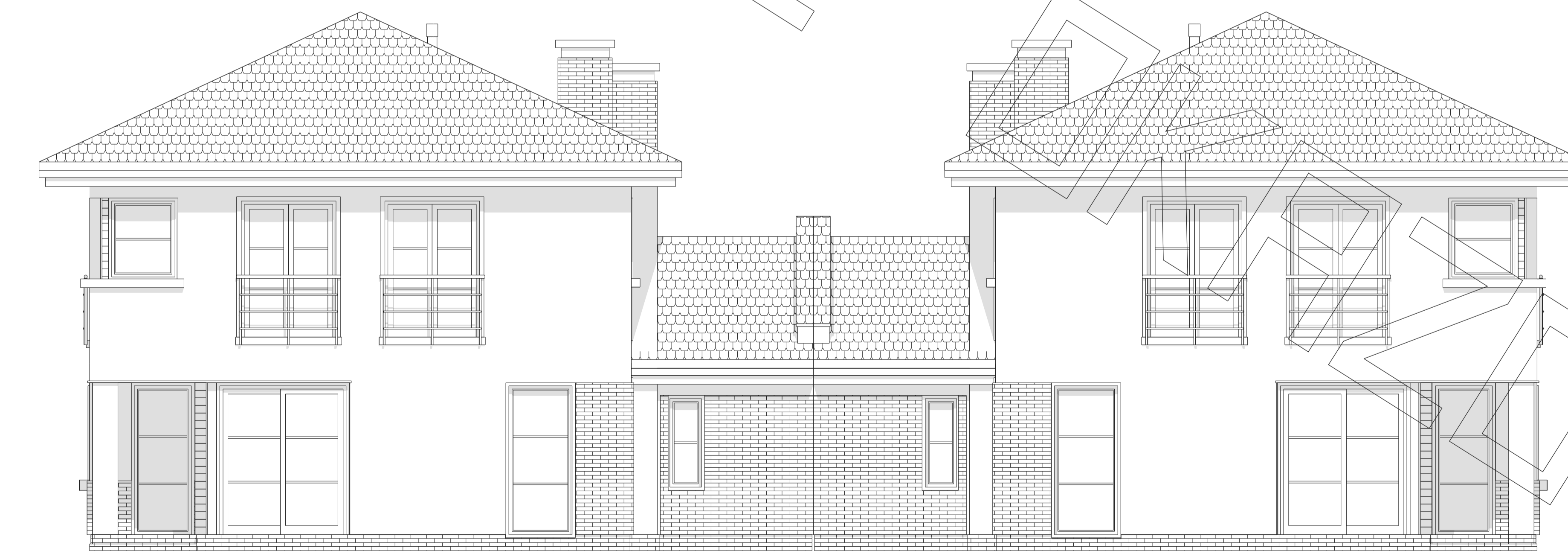
ELEWACJA TYLNA
