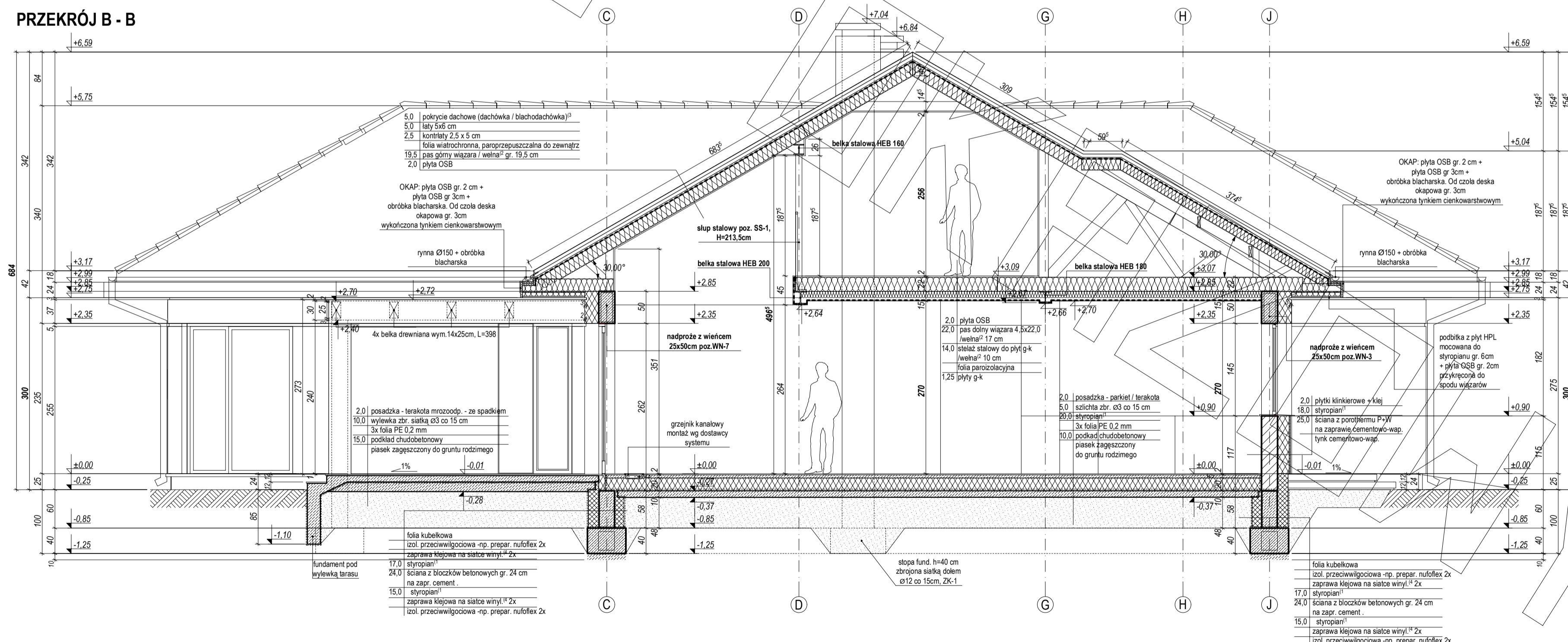
PRZEKRÓJ B - B
