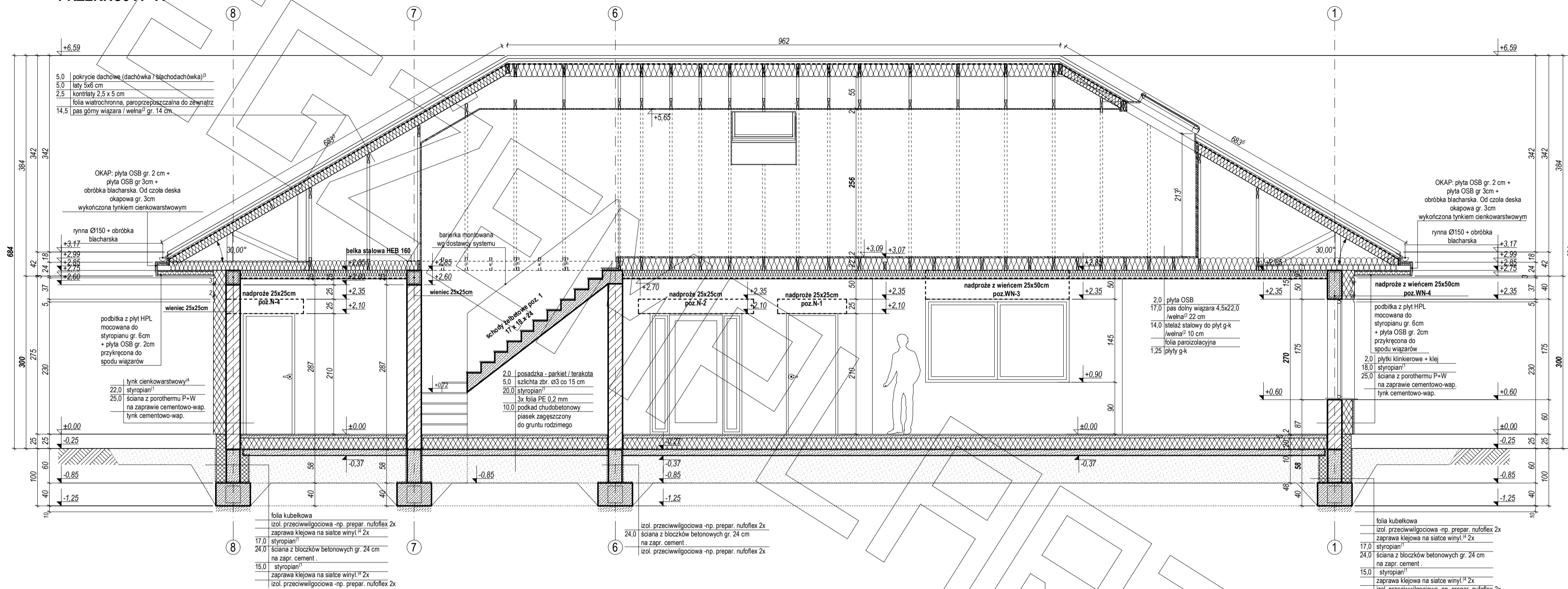
PRZEKRÓJ A - A
