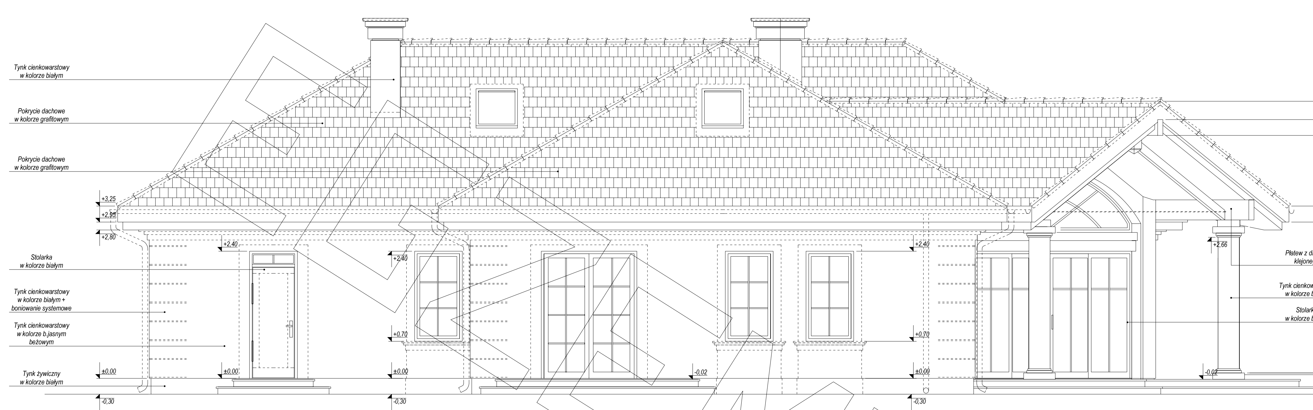
ELEWACJA TYLNA
