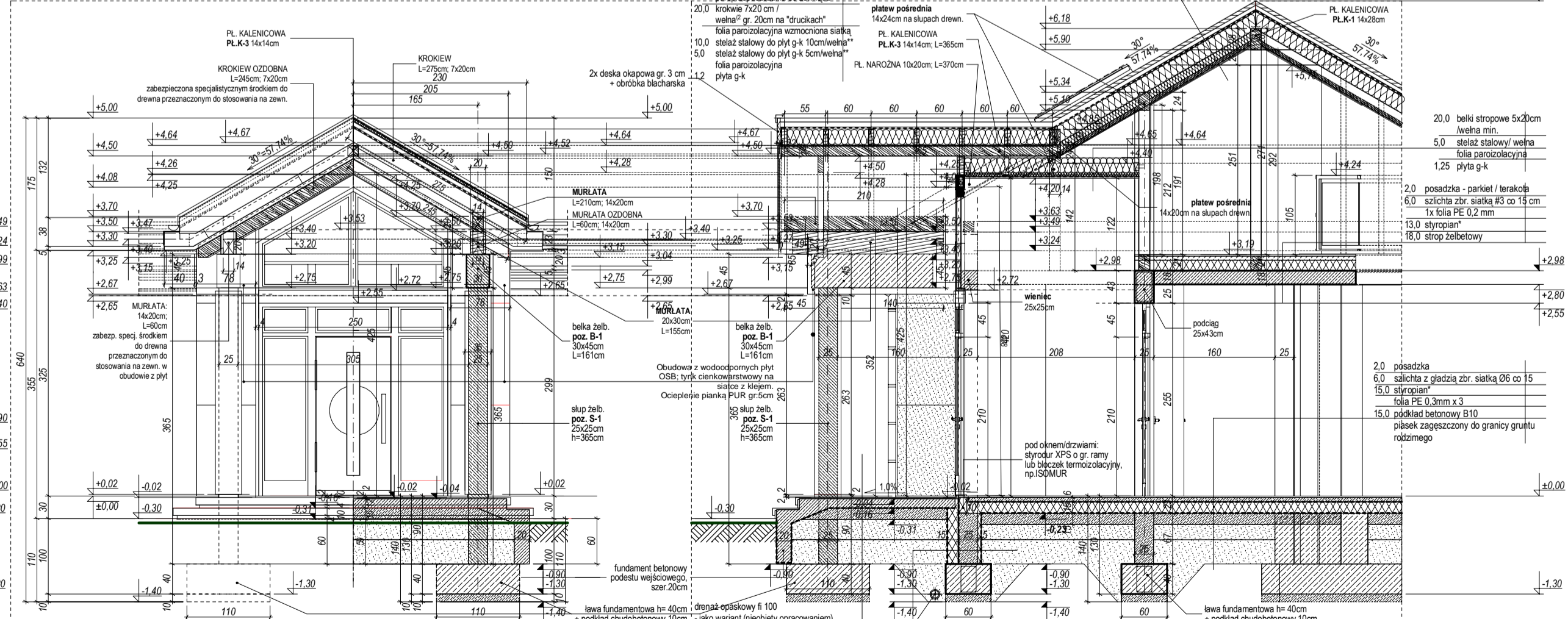
PRZEKRÓJ CC
