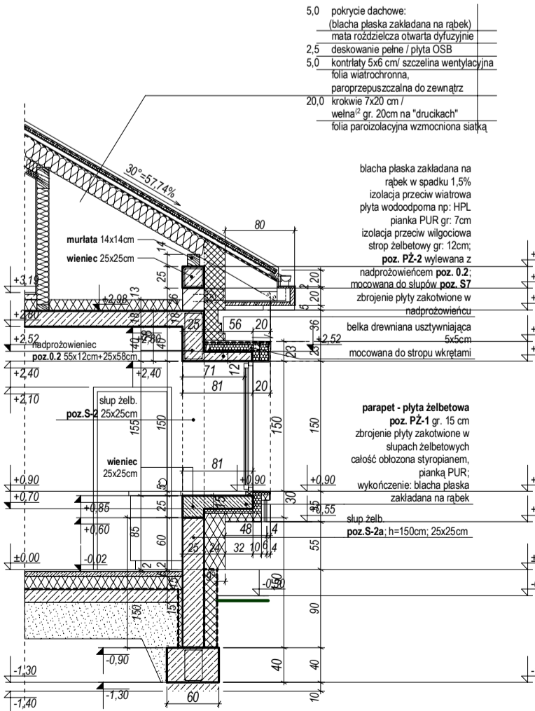
PRZEKRÓJ FF
