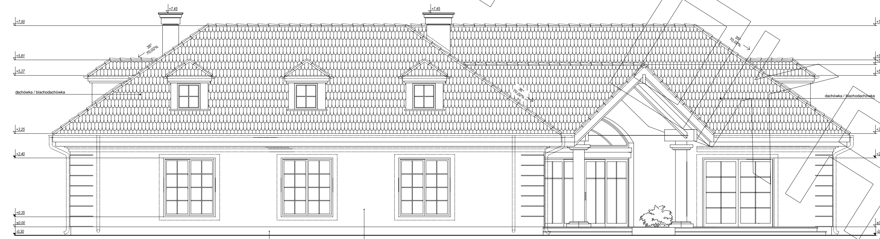
ELEWACJA BOCZNA
