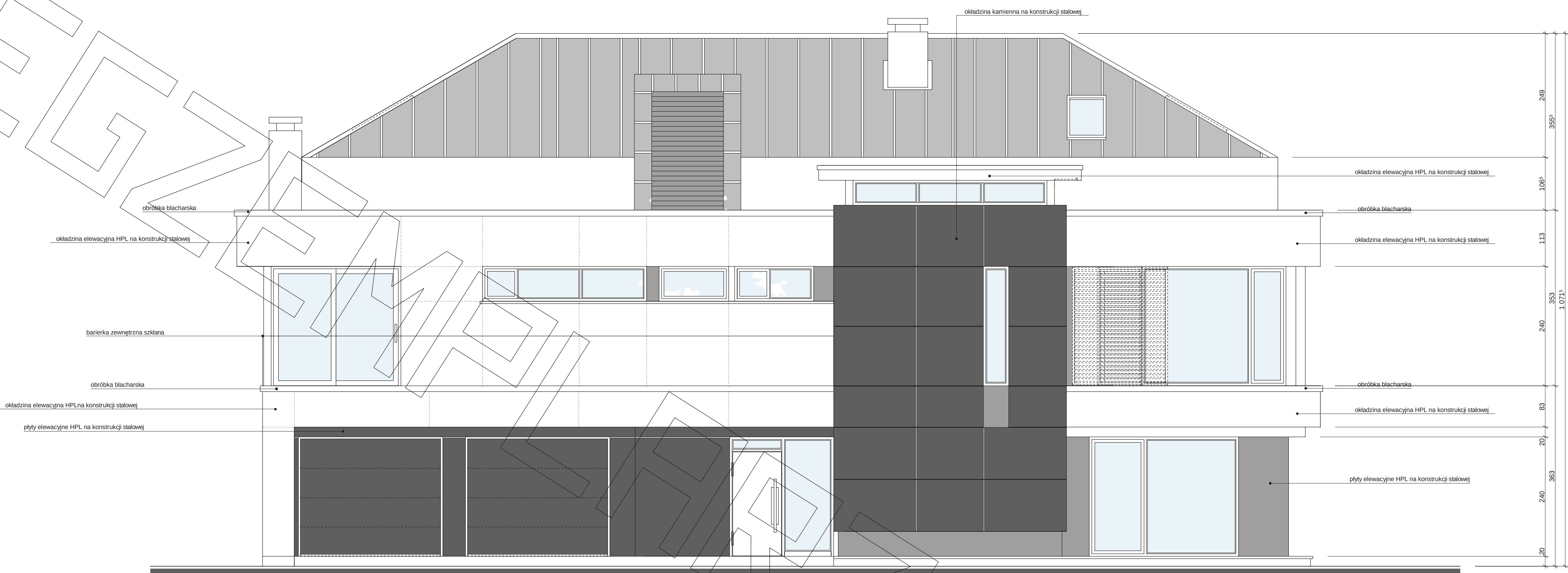
ELEWACJA FRONTOWA :
