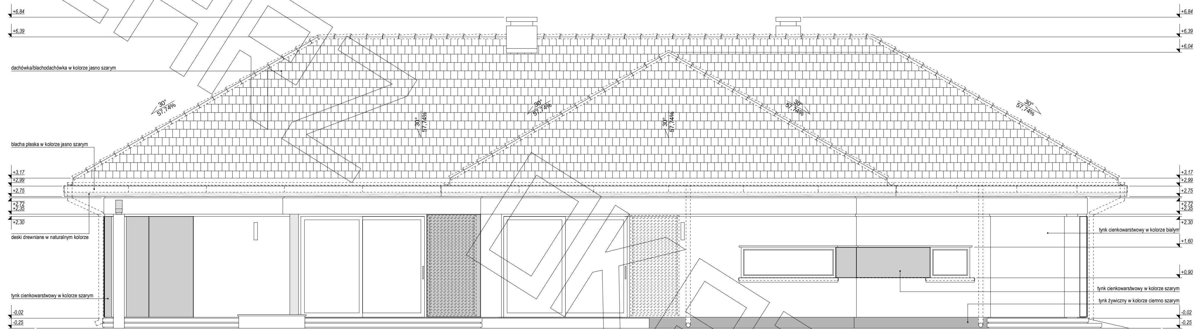
ELEWACJA BOCZNA:
