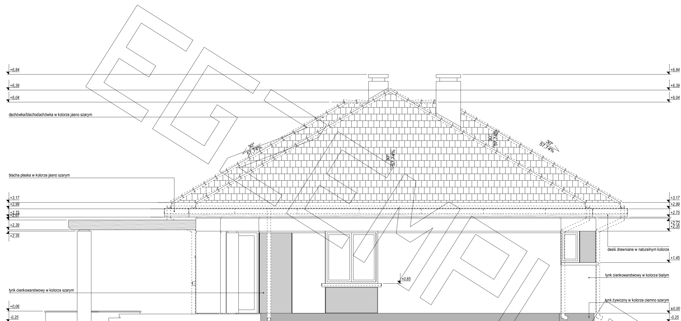
ELEWACJA TYLNA:
