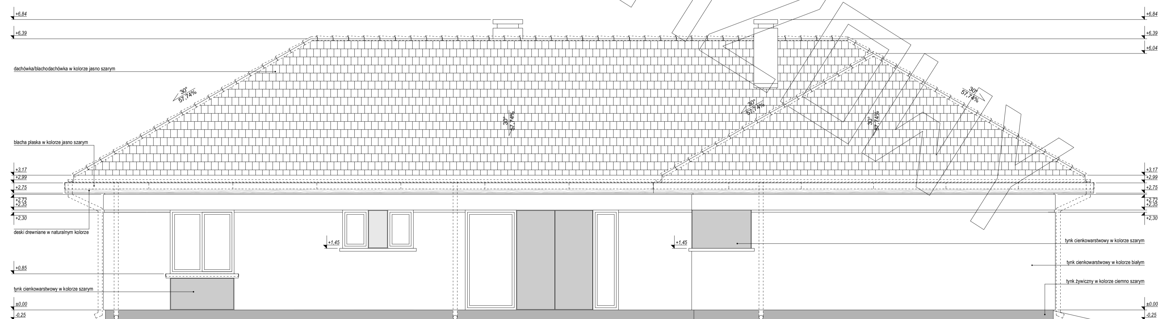
ELEWACJA BOCZNA:
