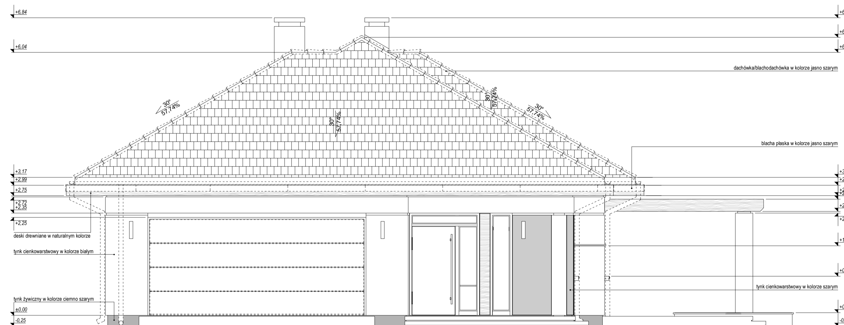
ELEWACJA FRONTOWA:
