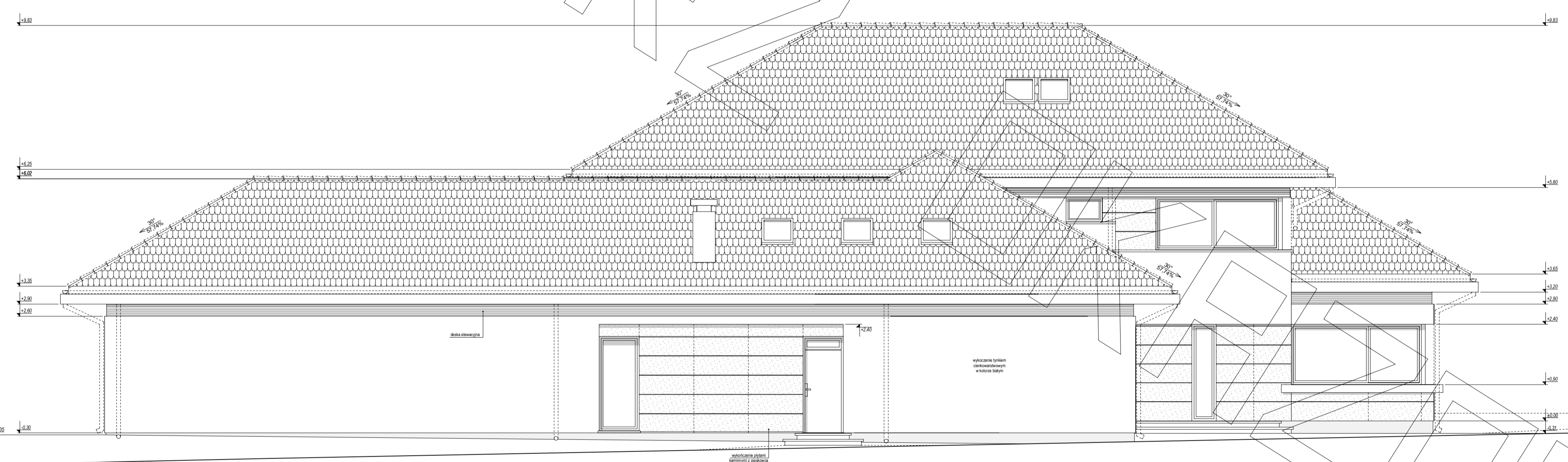
ELEWACJA BOCZNA
