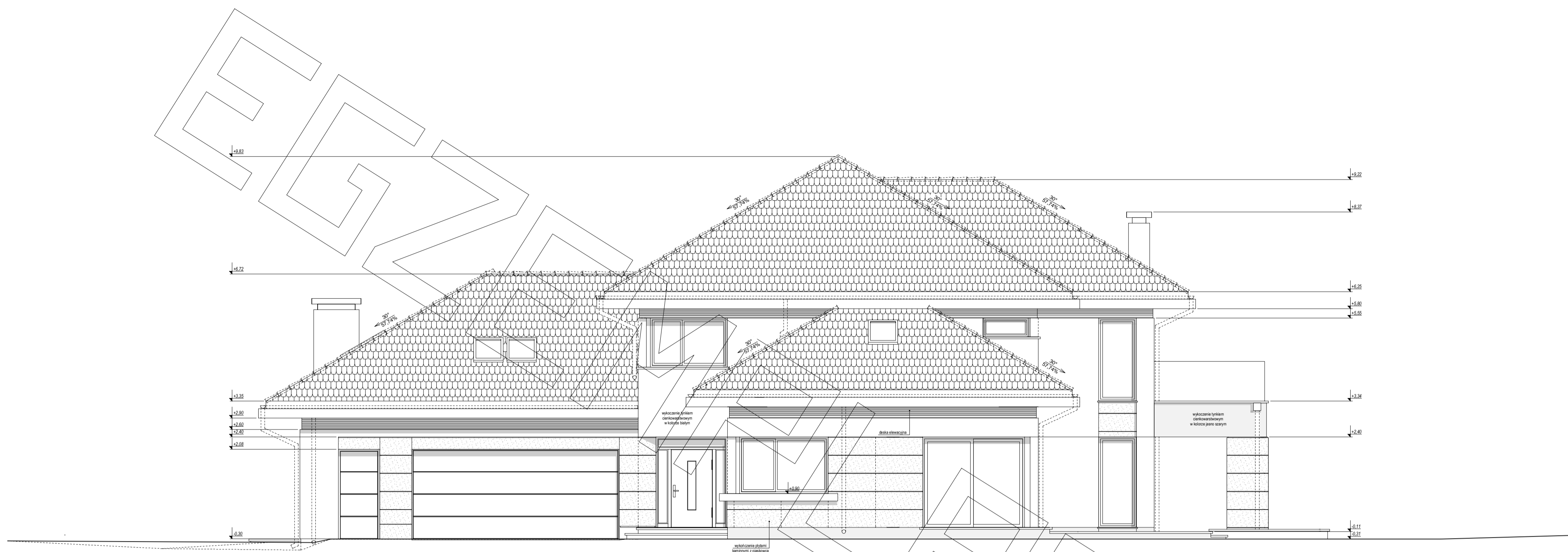
ELEWACJA FRONTOWA
