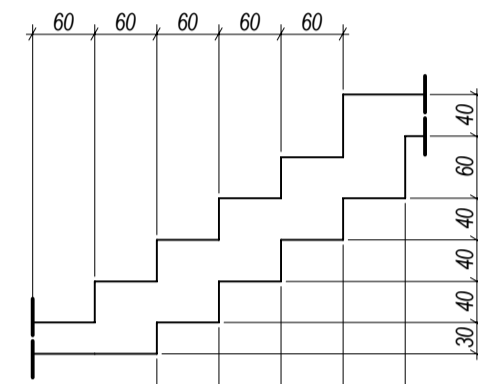
Wypycenie ławy fundamentowej
