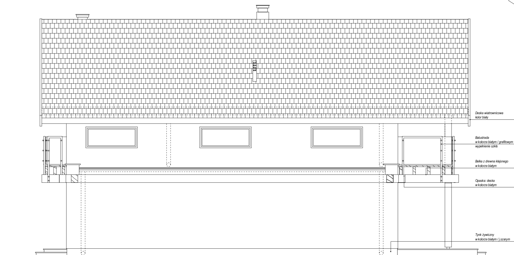
ELEWACJA BOCZNA
