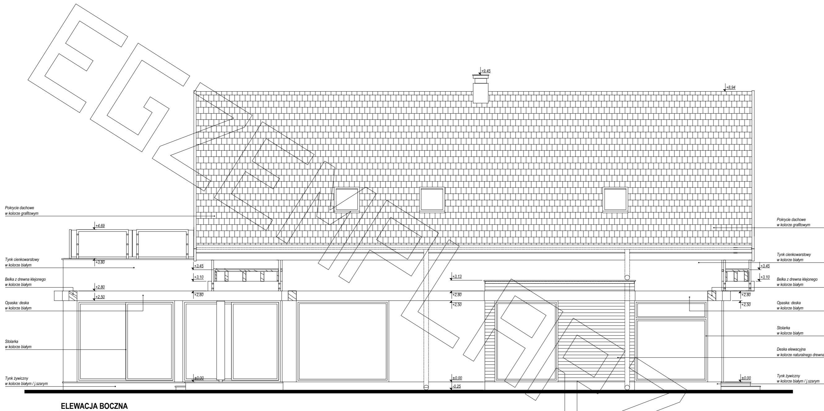
ELEWACJA BOCZNA
