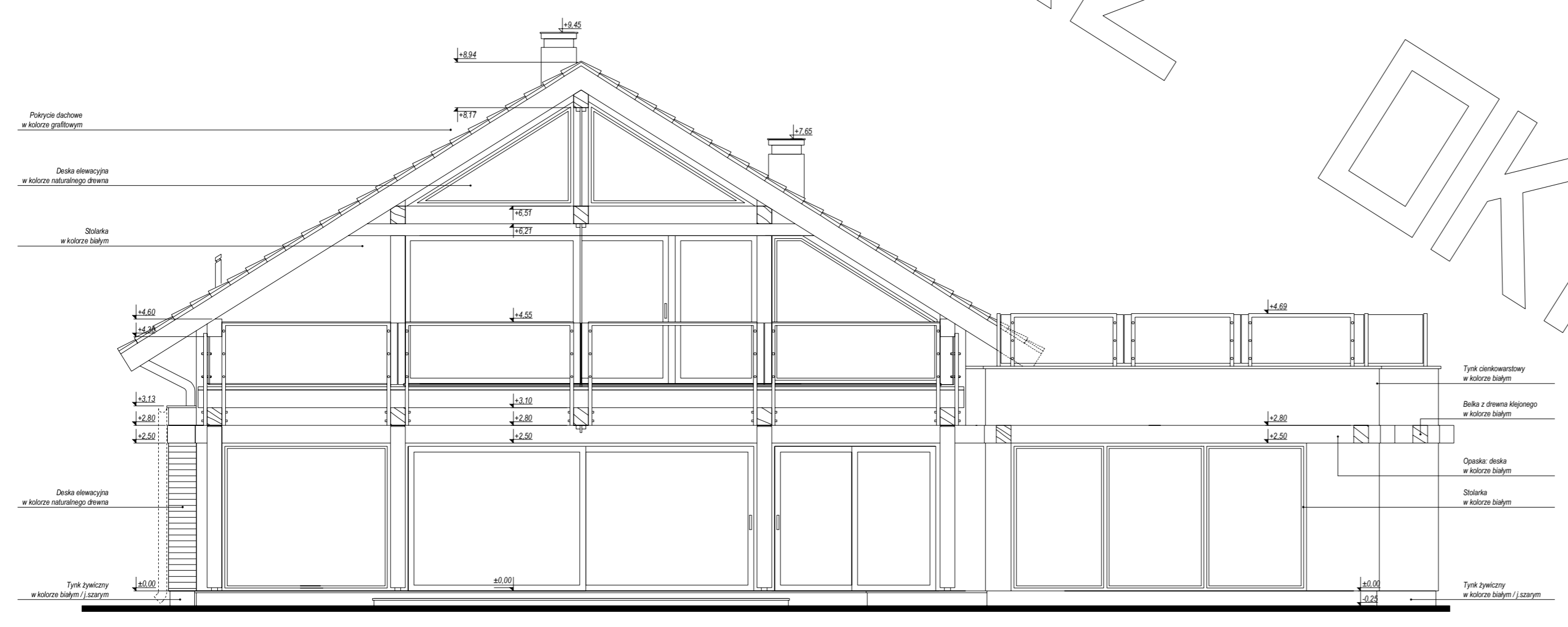
ELEWACJA TYLNA
