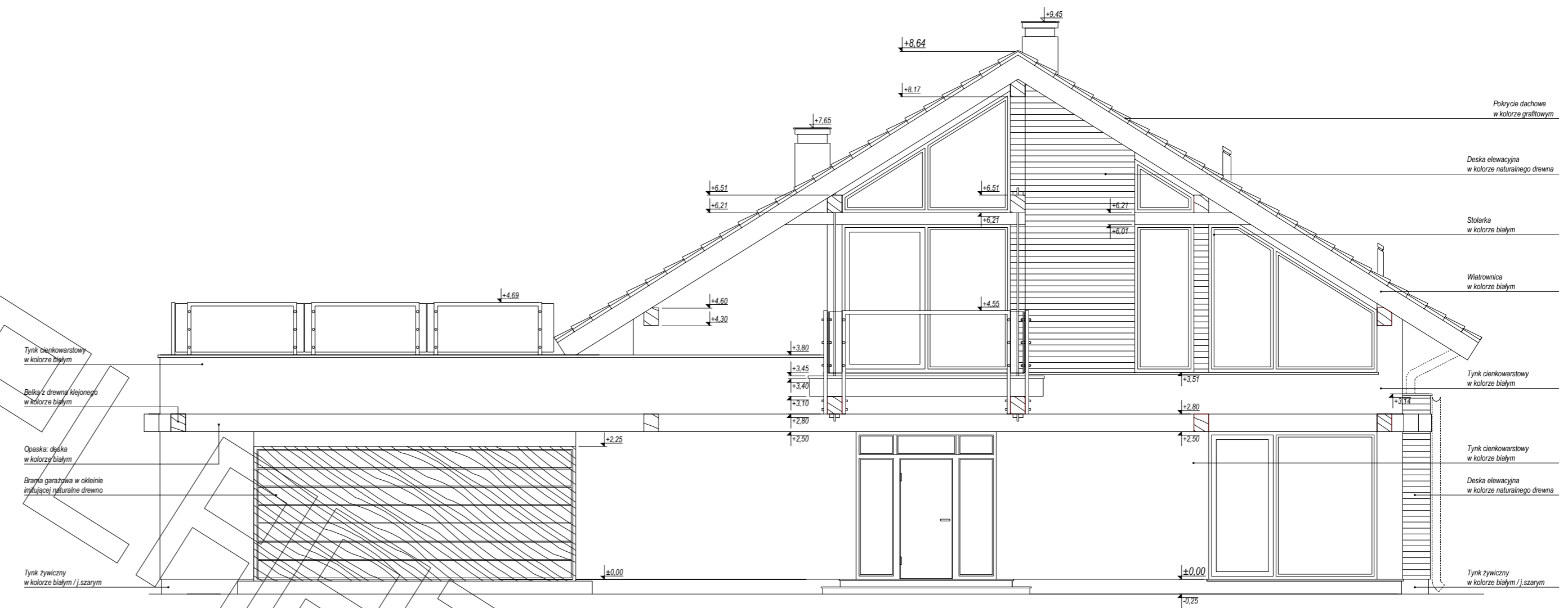
ELEWACJA FRONTOWA
