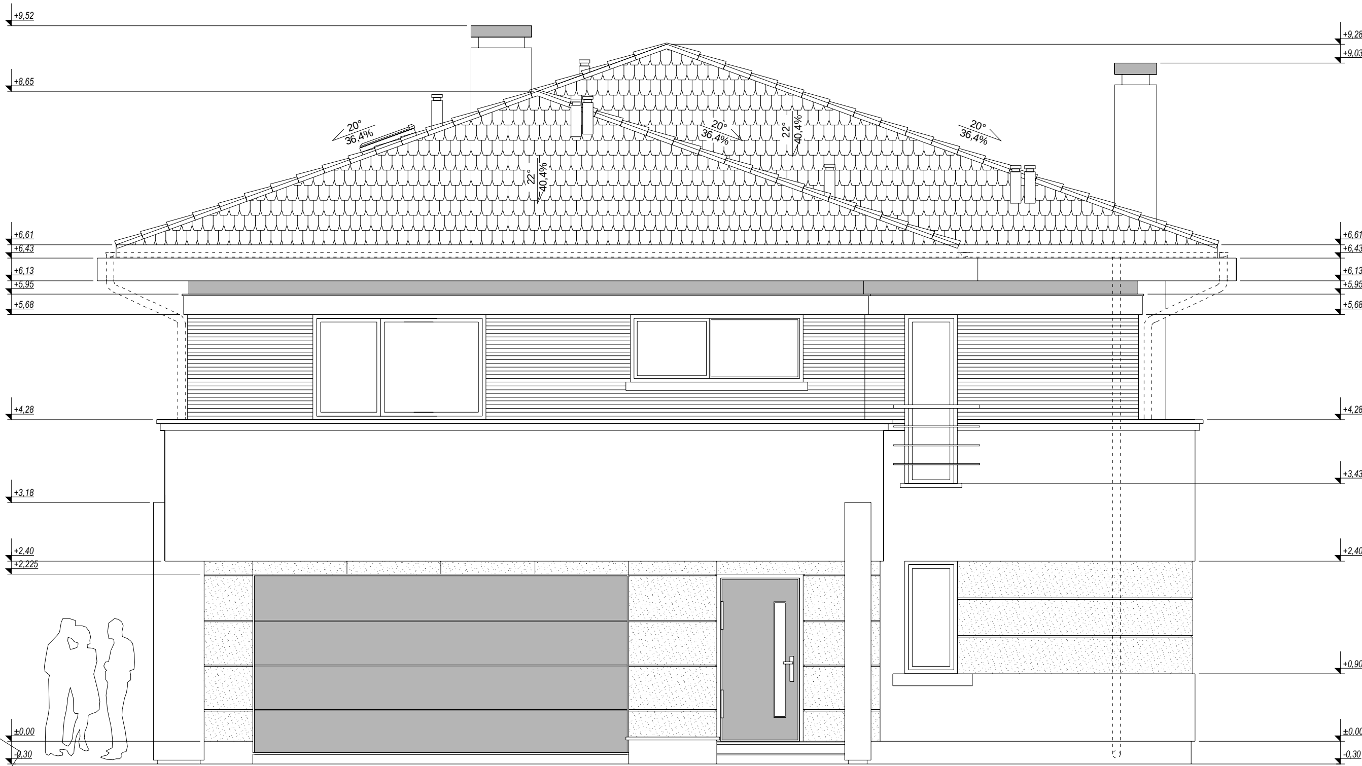
elewacja frontowa
