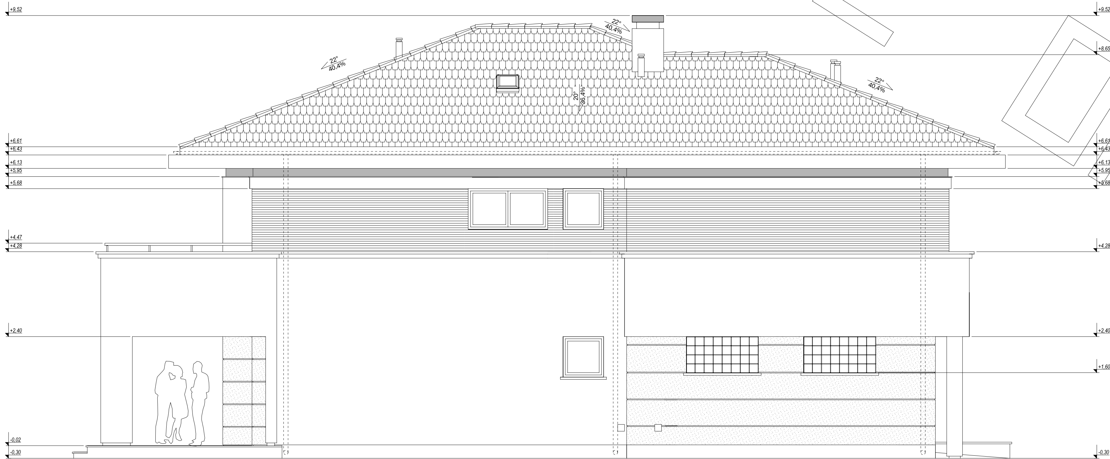
elewacja boczna
