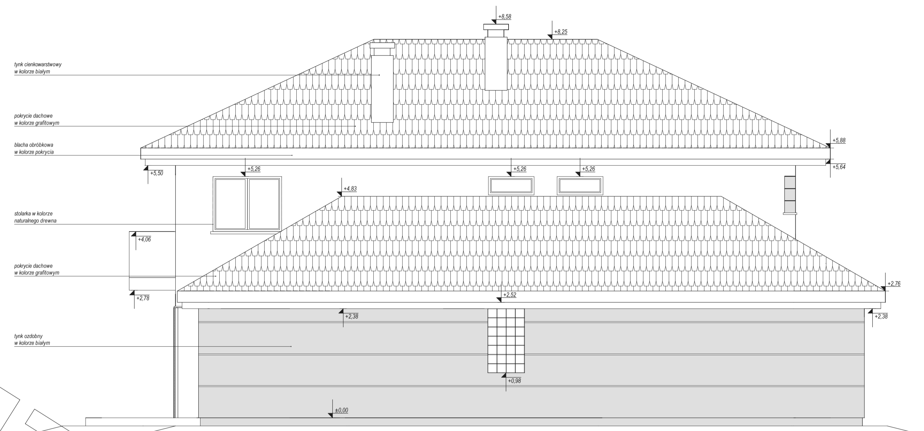
ELEWACJA BOCZNA
