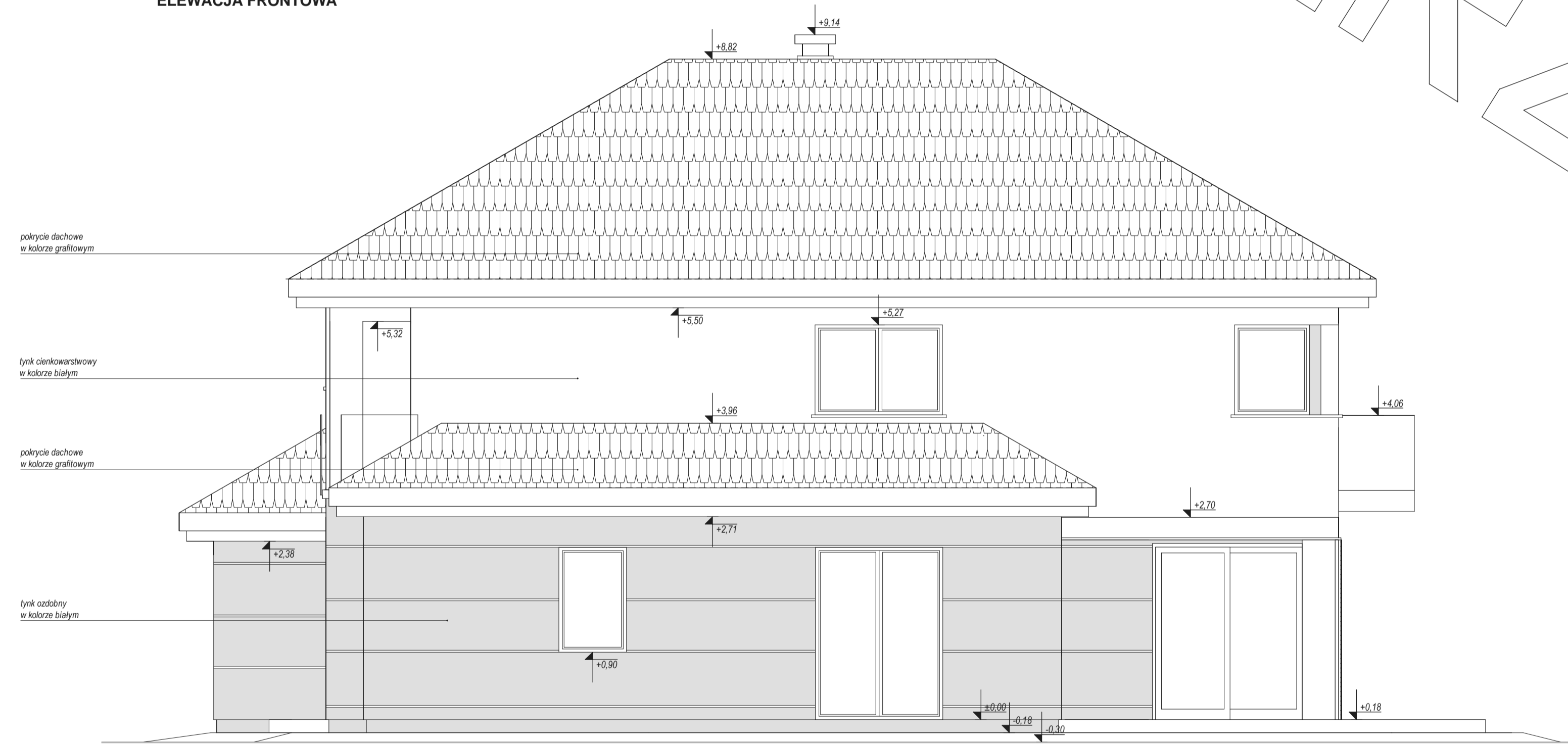
ELEWACJA BOCZNA
