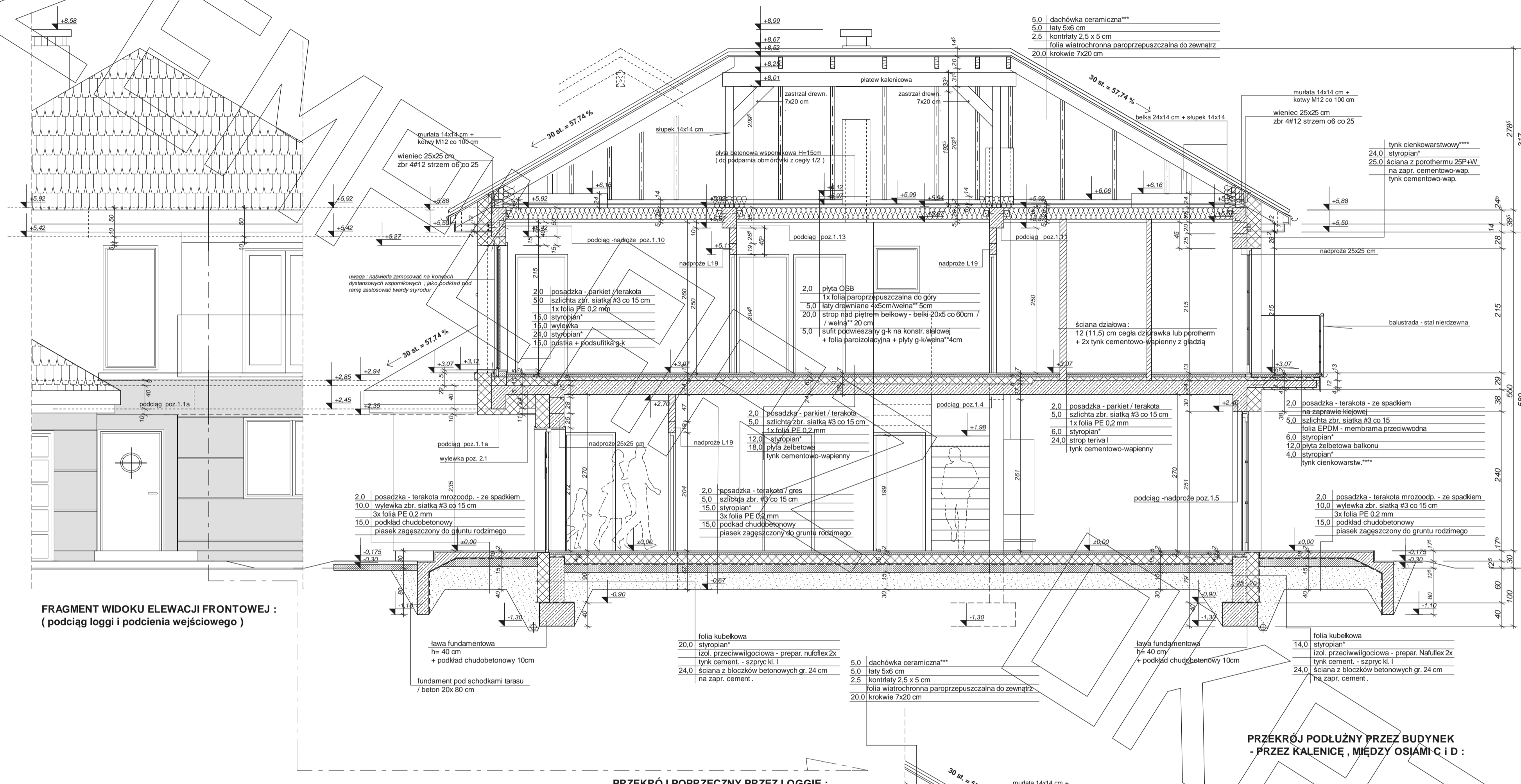
PRZEKRÓJ POPRZECZNY PRZEZ LOGGI :
