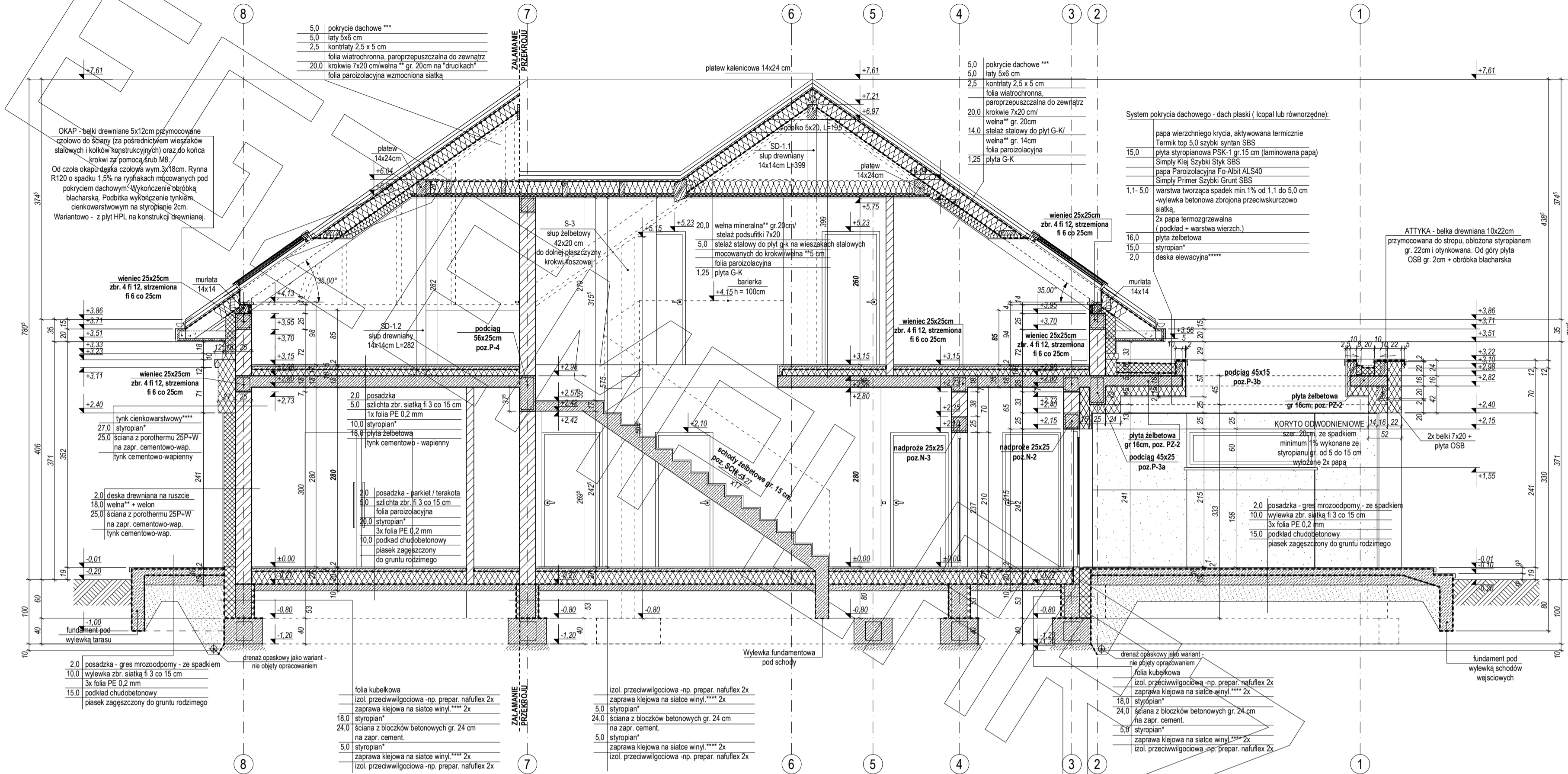
PRZEKRÓJ A-A
