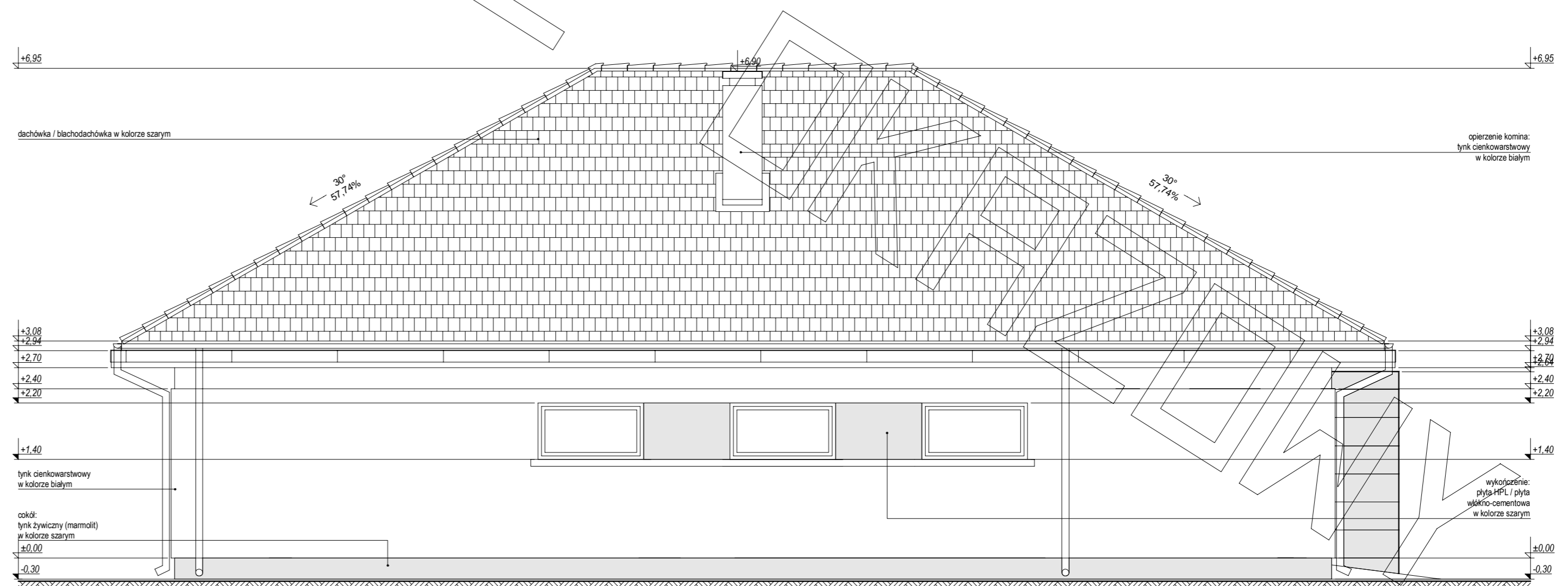
ELEWACJA BOCZNA:
