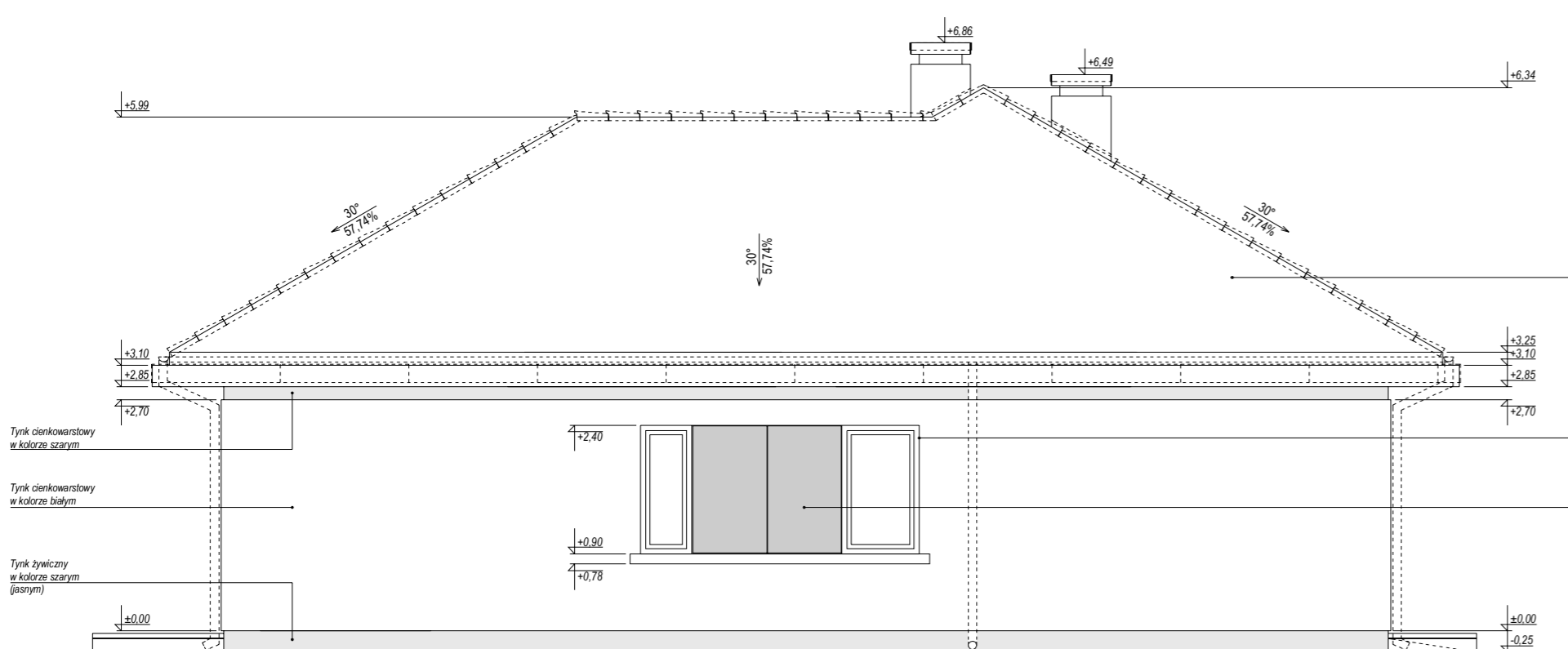
ELEWACJA BOCZNA
