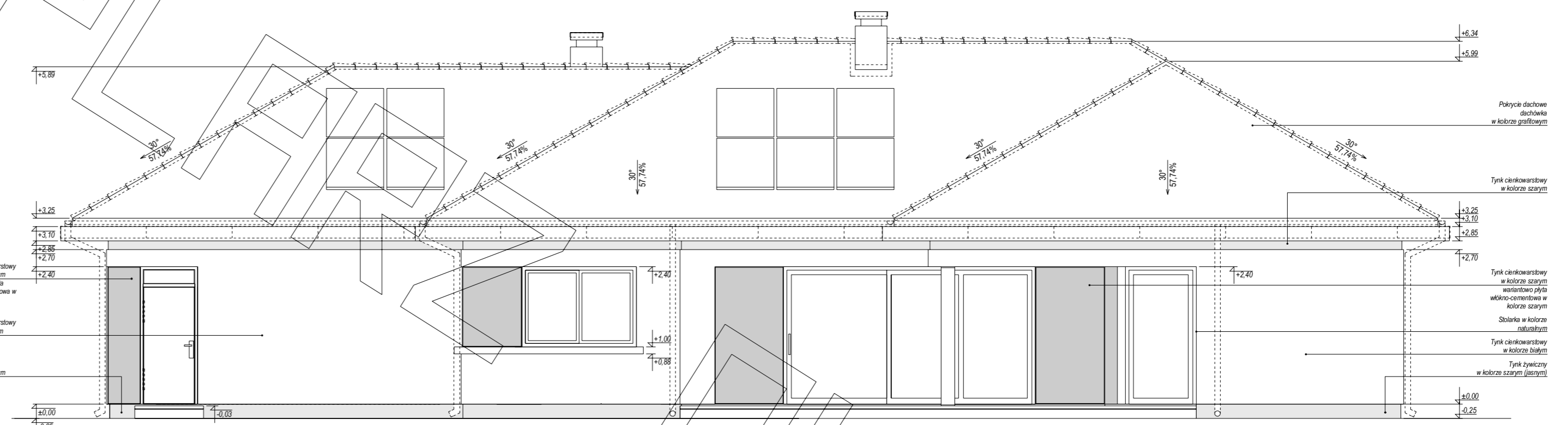
ELEWACJA TYLNA
