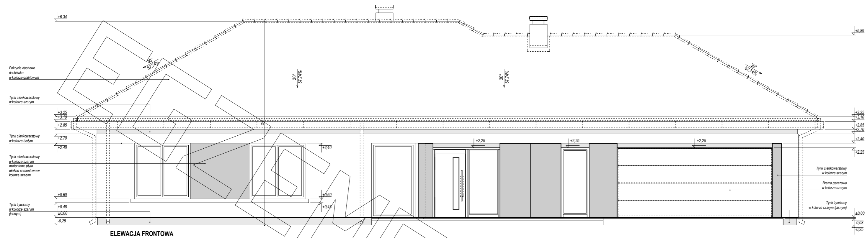
ELEWACJA FRONTOWA
