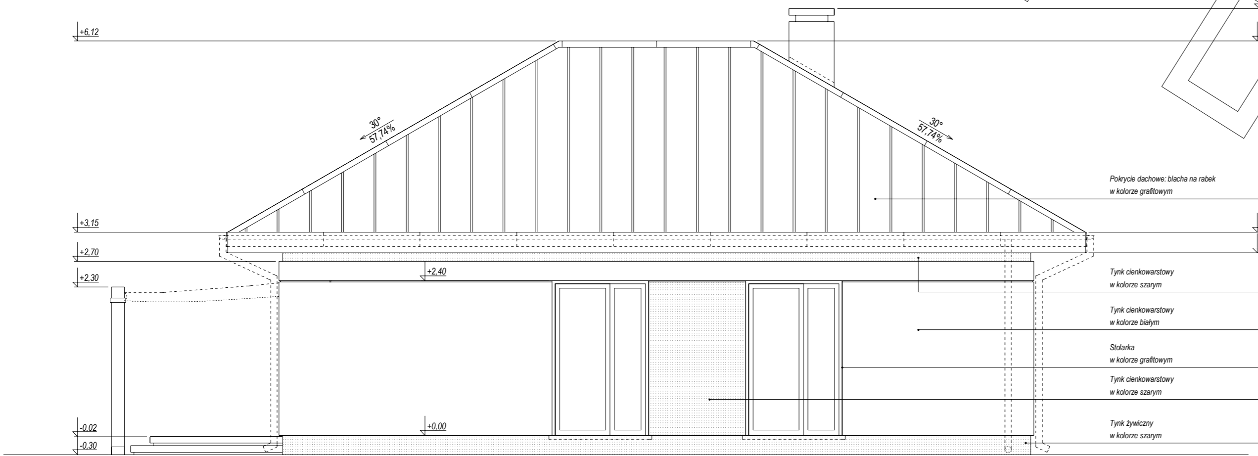
ELEWACJA TYLNA
