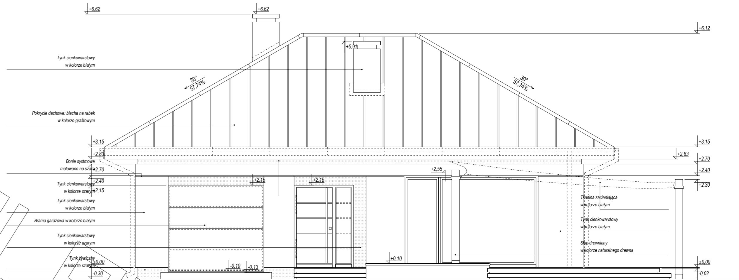
ELEWACJA FRONTOWA
