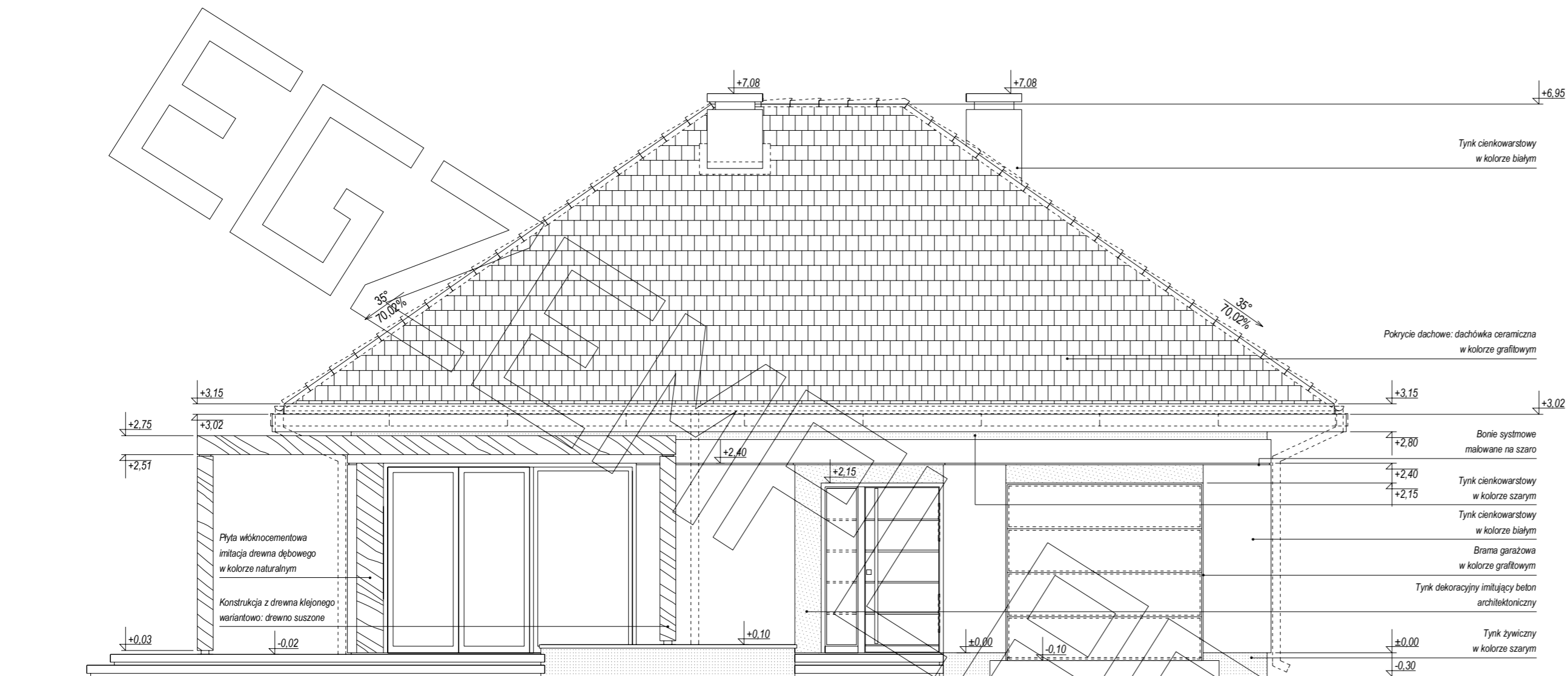
ELEWACJA FRONTOWA
