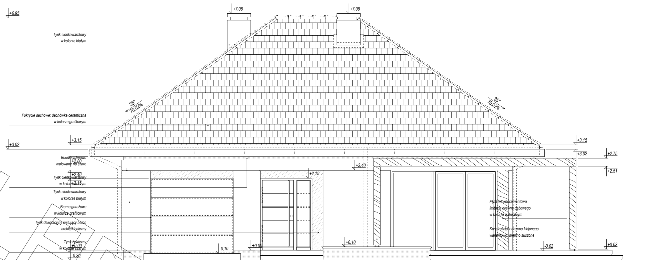
ELEWACJA FRONTOWA
