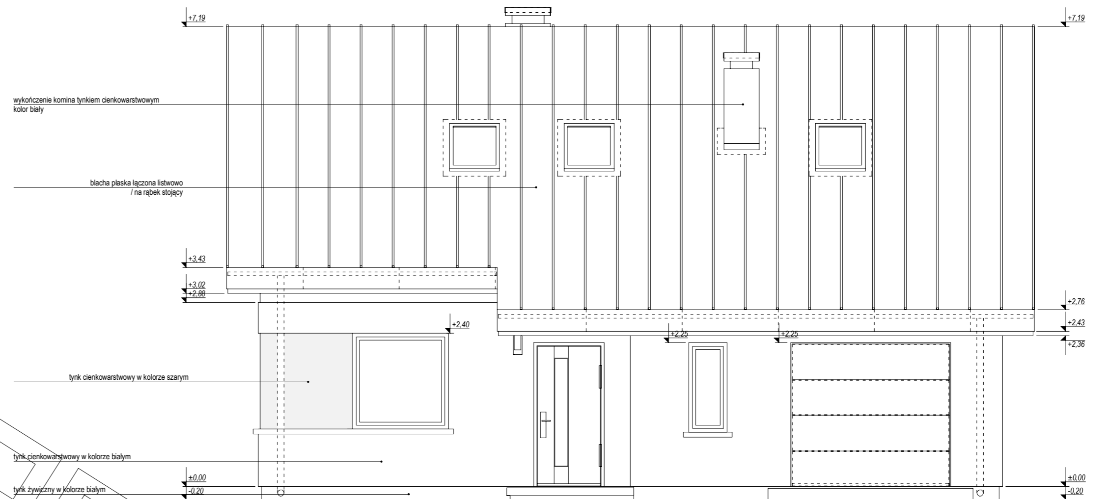
elewacja frontowa
