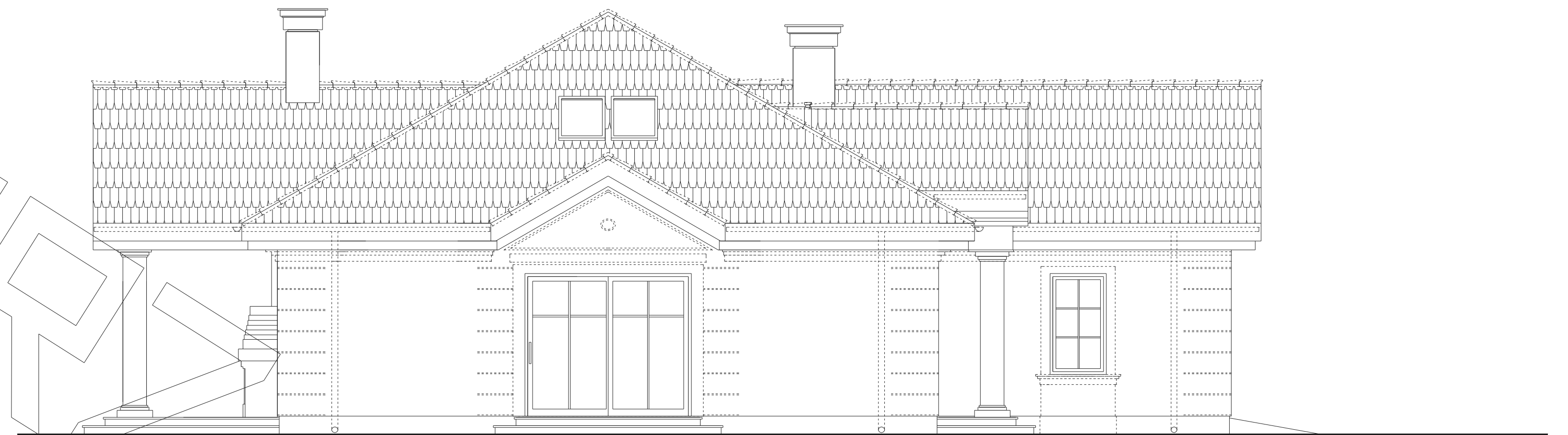
ELEWACJA BOCZNA
