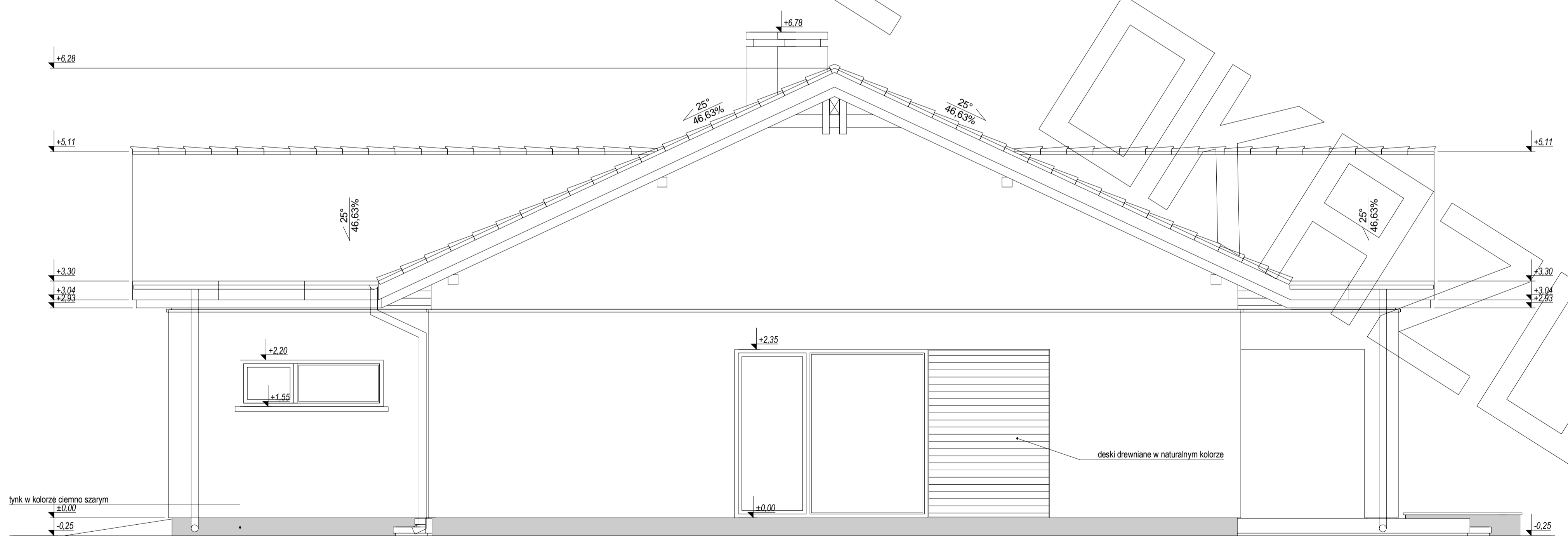
ELEWACJA BOCZNA:
