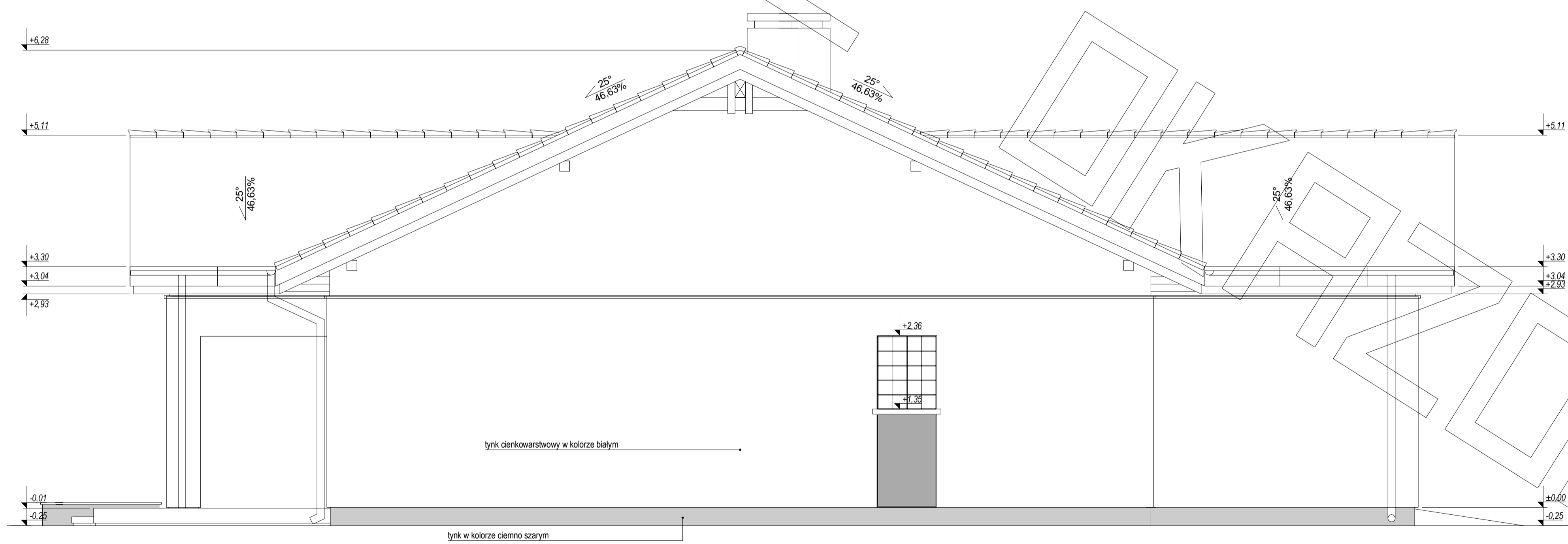
ELEWACJA BOCZNA:
